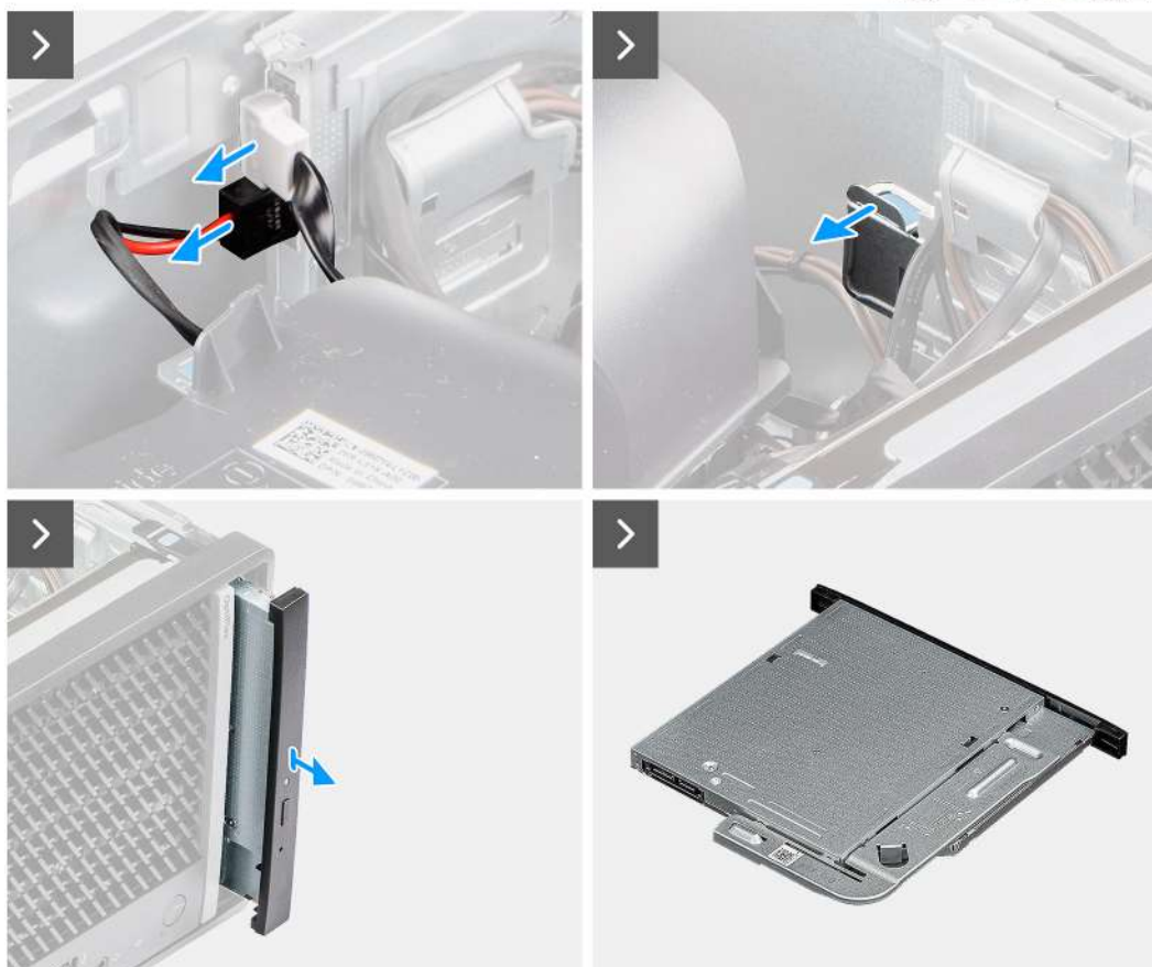
Obrázek 37. Demontáž tenké optické jednotky
