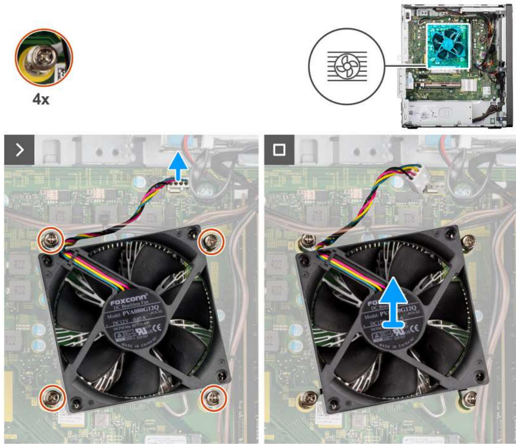
Obrázek 62. Demontáž sestavy ventilátoru procesoru a chladiče
