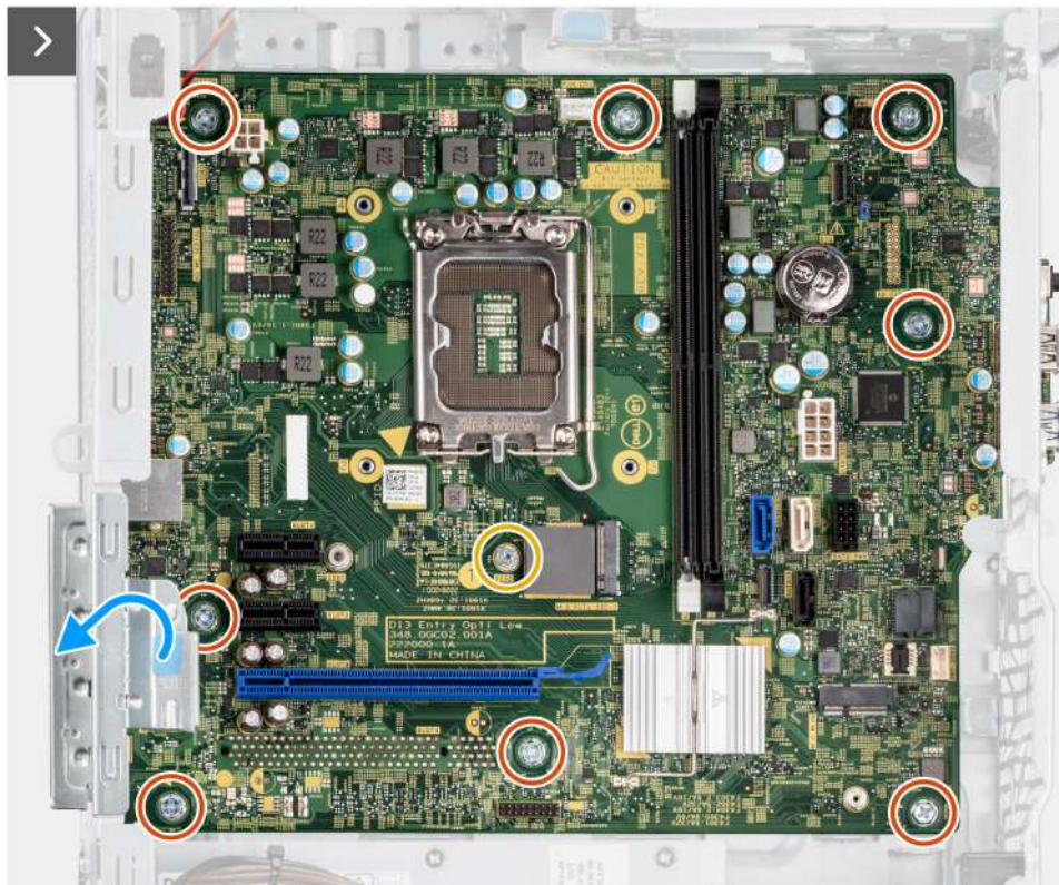
Obrázek 85. Demontáž základní desky
