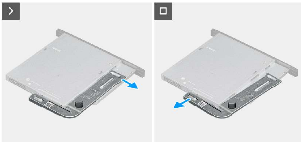
Obrázek 38. Demontáž tenké optické jednotky
