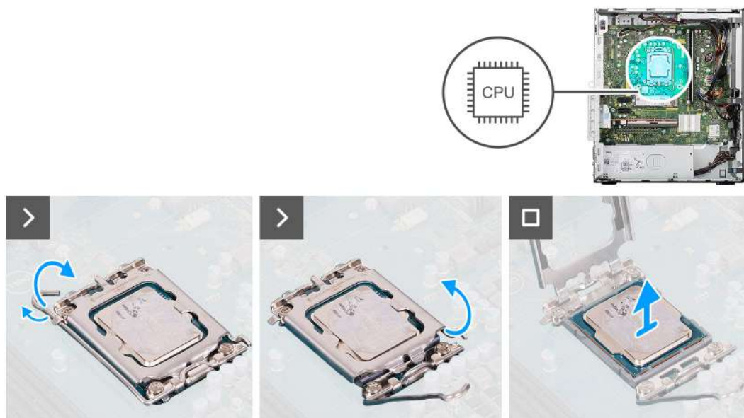
Obrázek 68. Demontáž procesoru
