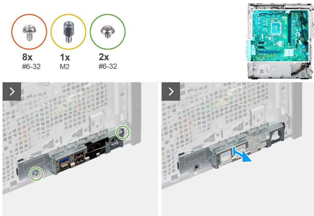
Obrázek 83. Demontáž základní desky
