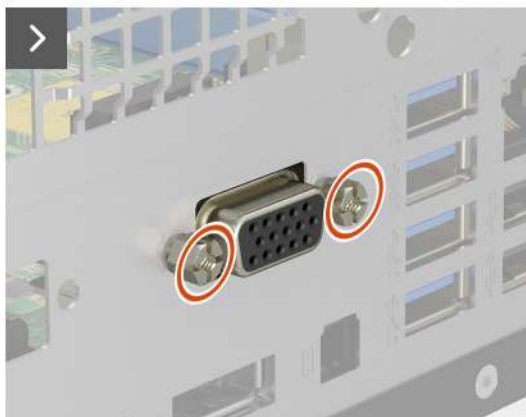
Obrázek 80. Demontáž volitelného modulu VGA
