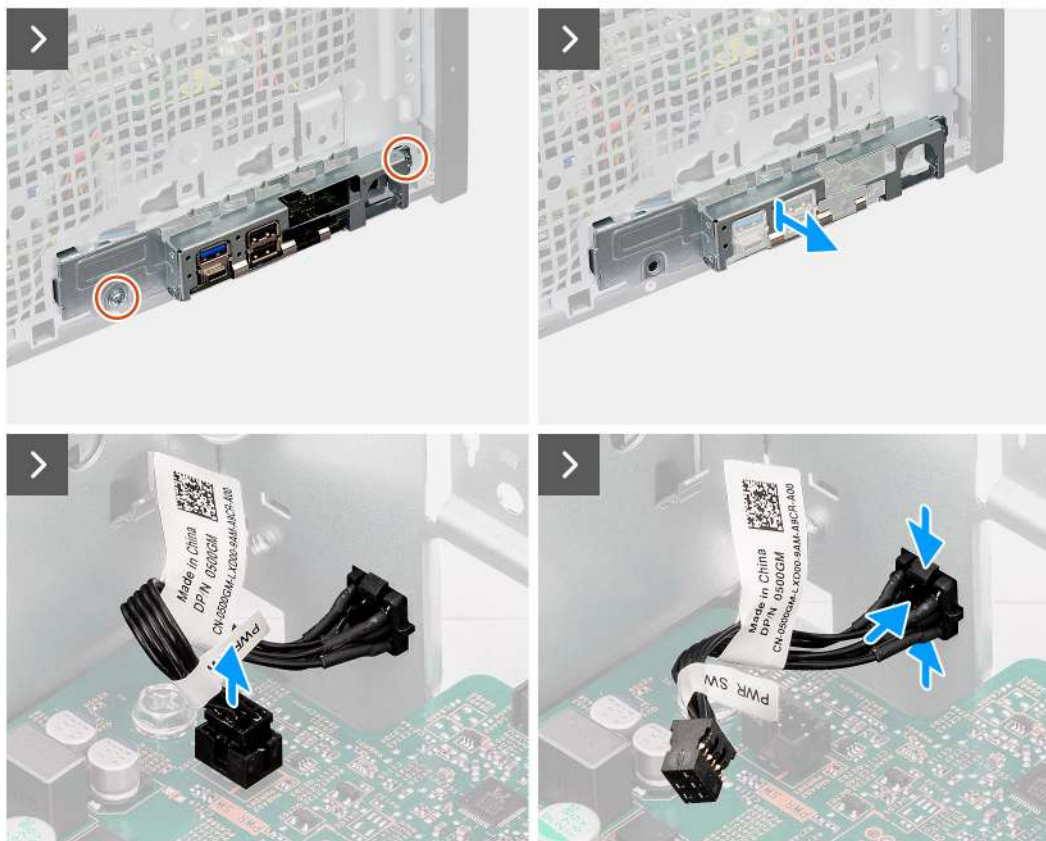
Obrázek 49. Demontáž vypínače
