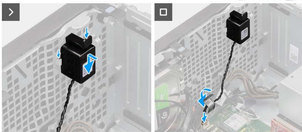
Obrázek 42. Montáž interního reproduktoru
