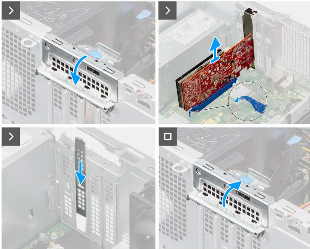
Obrázek 33. Demontáž grafické karty
