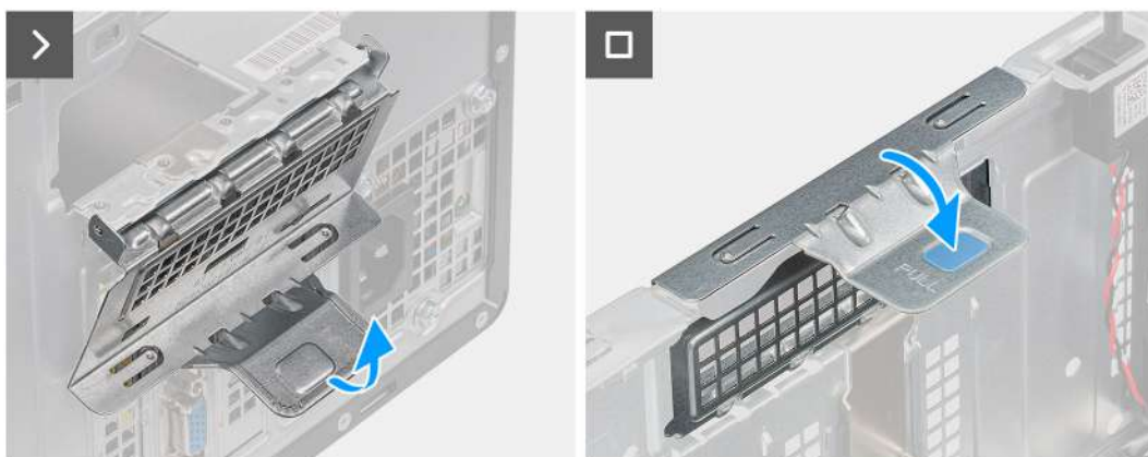
Obrázek 46. Montáž karty sériového/paralelního portu
