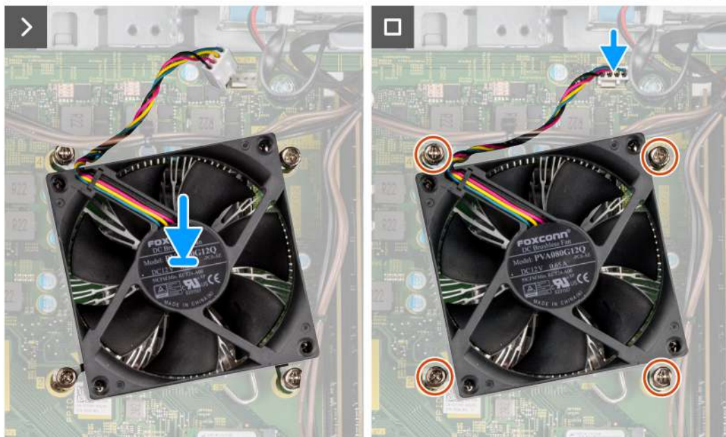
Obrázek 63. Montáž sestavy ventilátoru a chladiče procesoru
