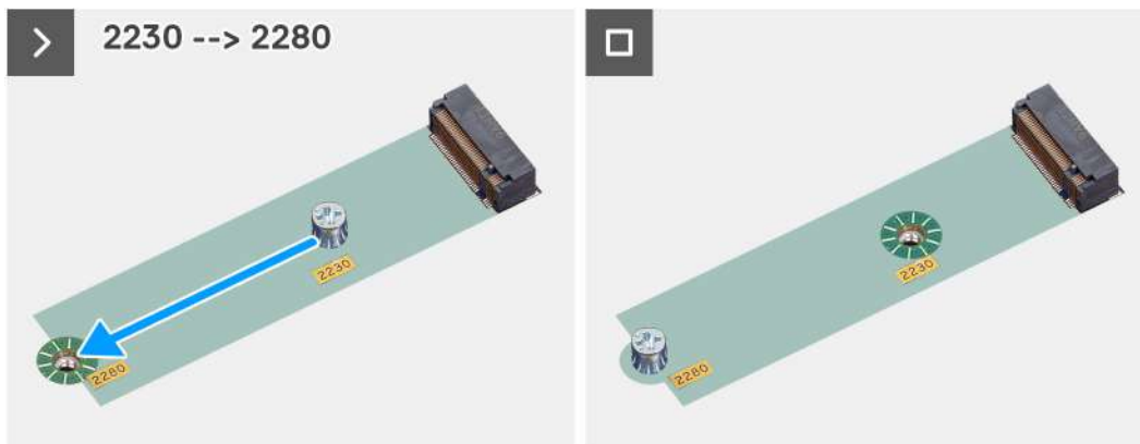
Obrázek 23. Montáž disku SSD M.2 2230
