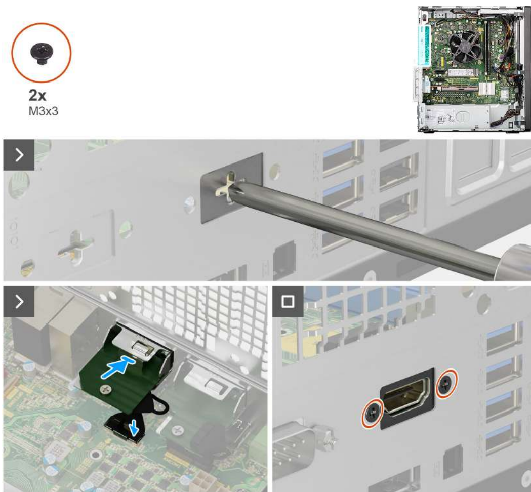
Obrázek 77. Montáž volitelného modulu HDMI
