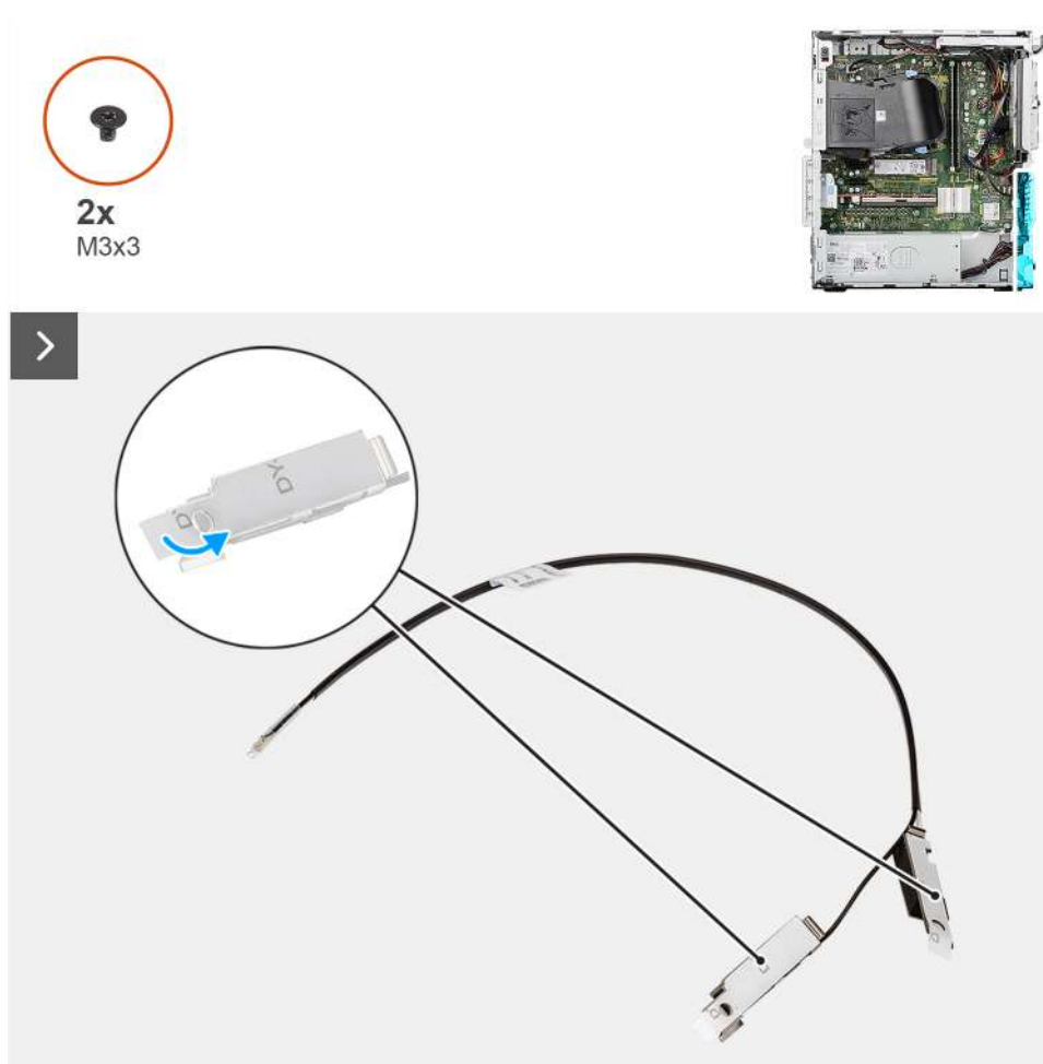
Obrázek 54. Montáž modulu interní antény
