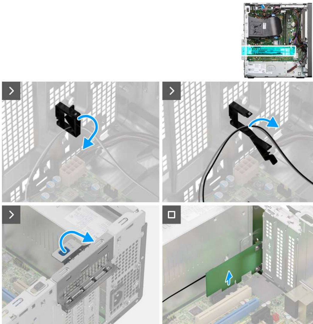
Obrázek 56. Demontáž modulu externí antény SMA
