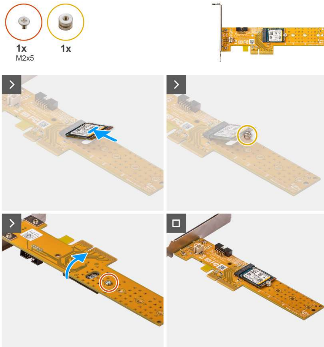
Obrázek 28. Montáž karty Dell Ultra Speed 3. generace s diskem M.2 2230
