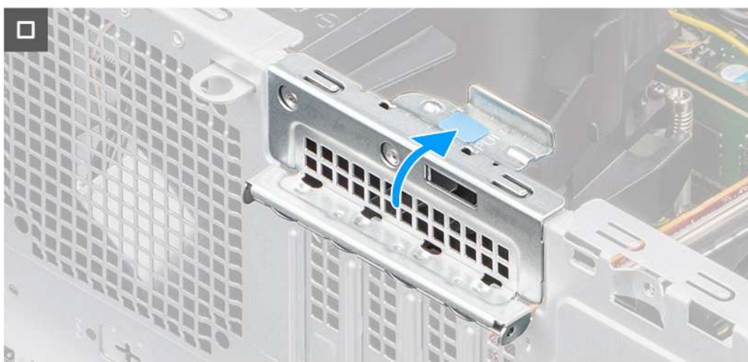
Obrázek 75. Montáž volitelného modulu PS2 a sériového modulu
