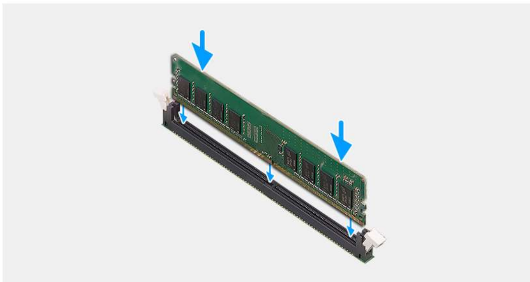
Obrázek 18. Vložení paměťového modulu
