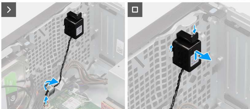
Obrázek 41. Demontáž interního reproduktoru
