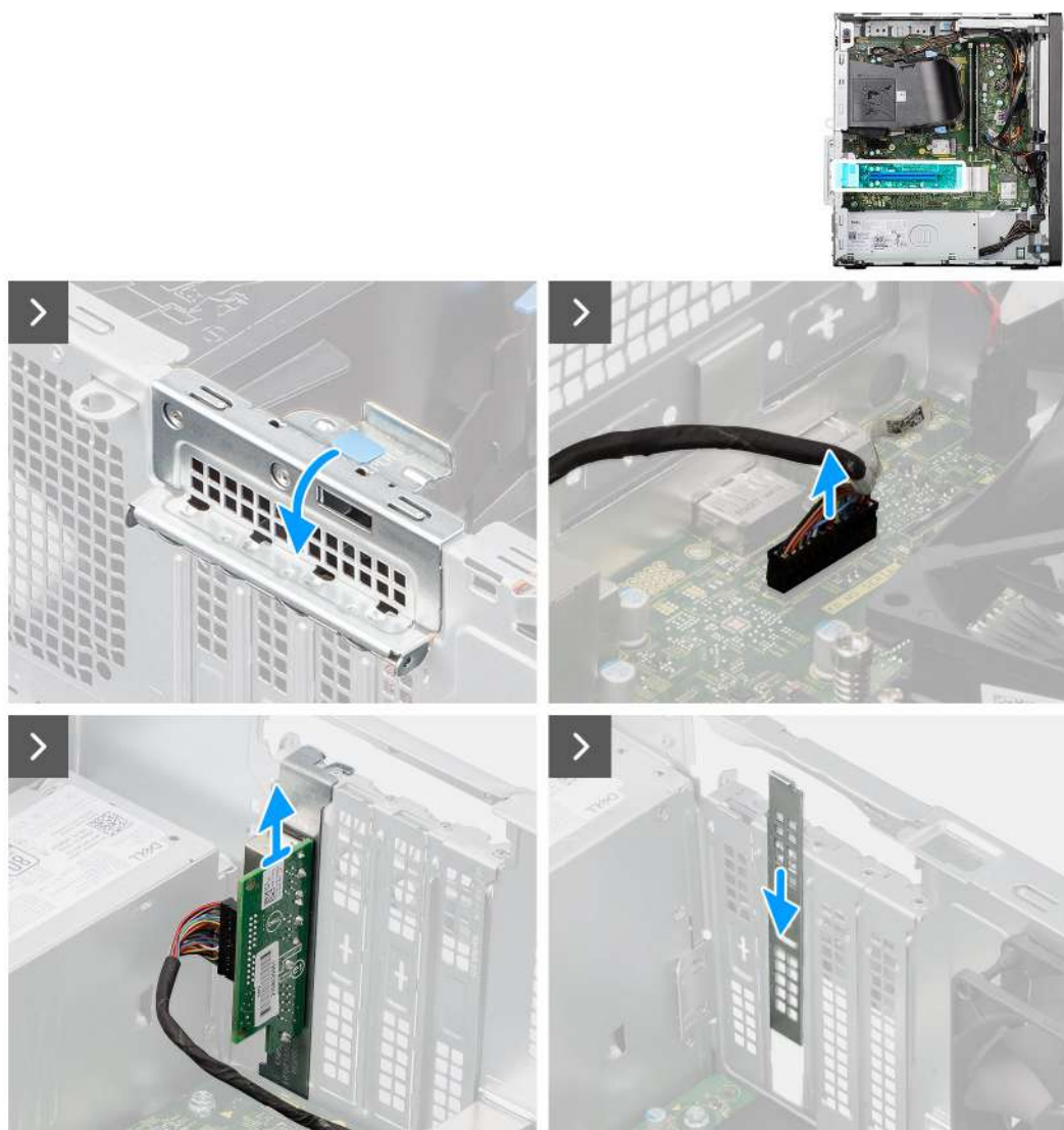
Obrázek 72. Demontáž volitelného modulu PS2 a sériového modulu
