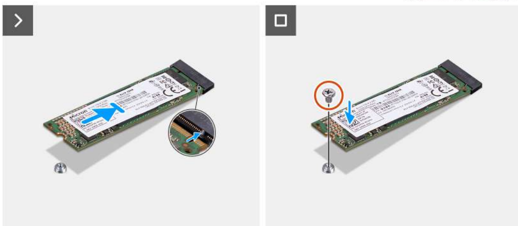
Obrázek 24. Montáž disku SSD M.2 2280
