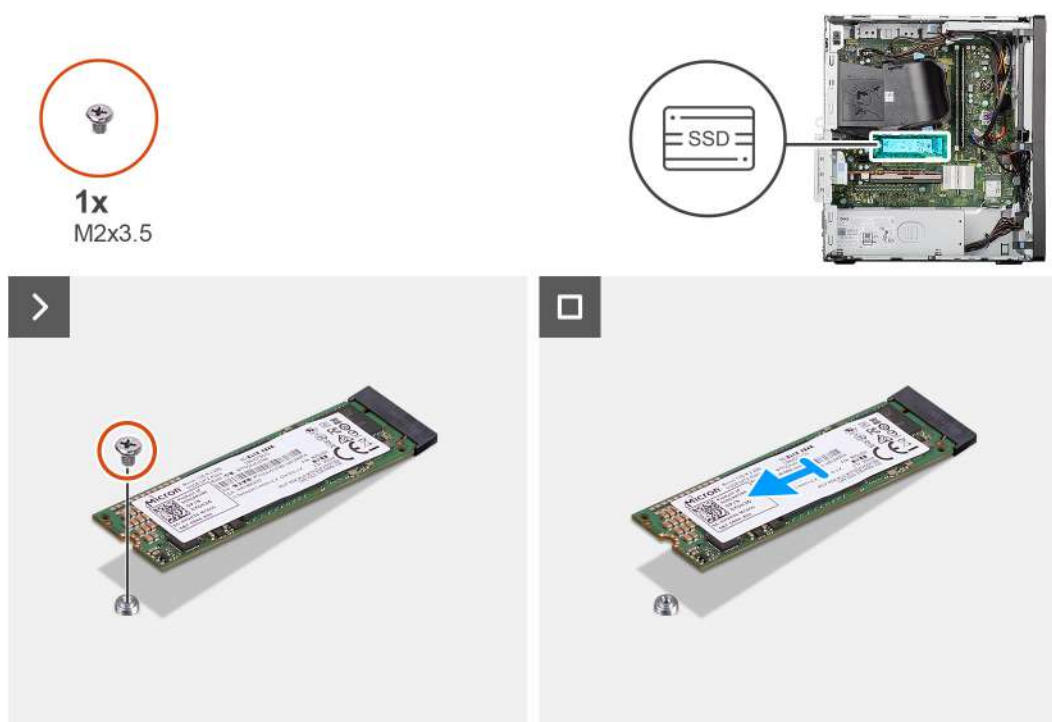
Obrázek 22. Demontáž disku SSD M.2 2280
