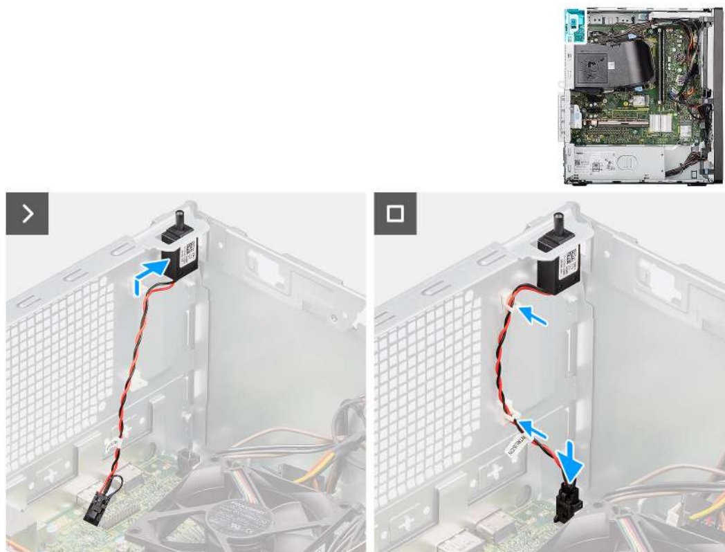
Obrázek 48. Montáž spínače detekce vniknutí do šasi
