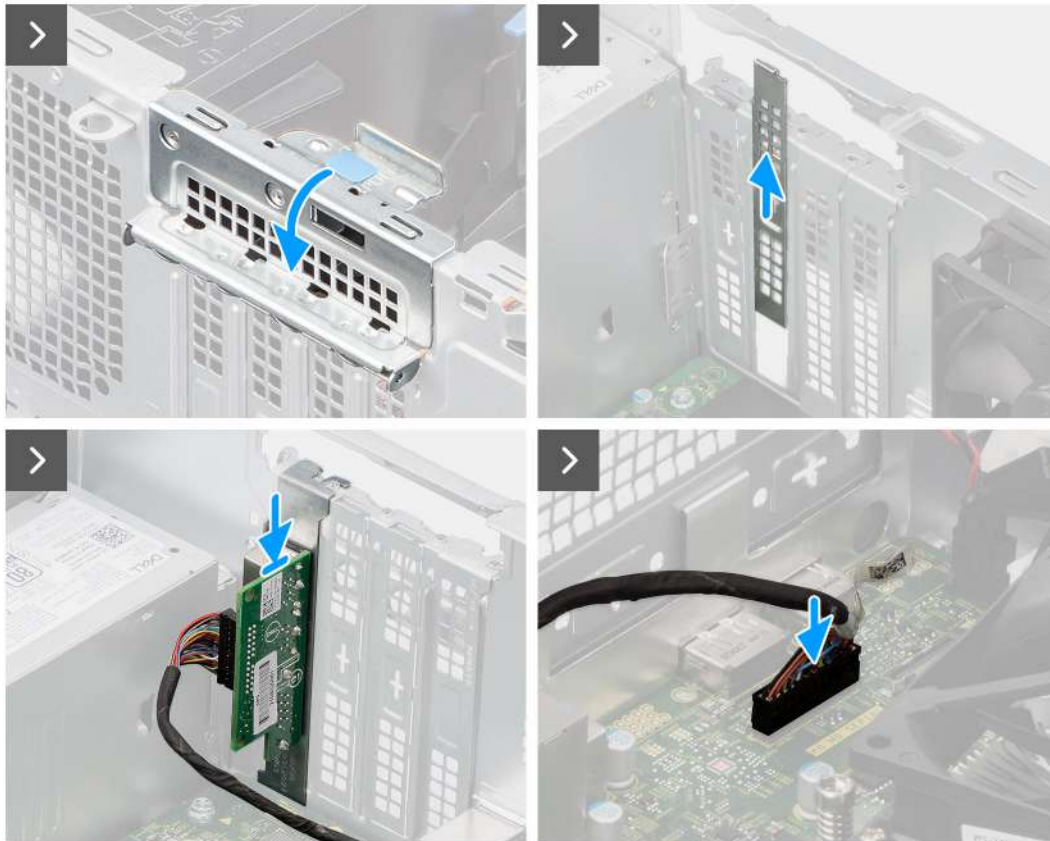
Obrázek 74. Montáž volitelného modulu PS2 a sériového modulu
