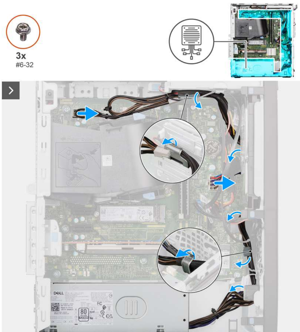
Obrázek 64. Demontáž napájecí jednotky
