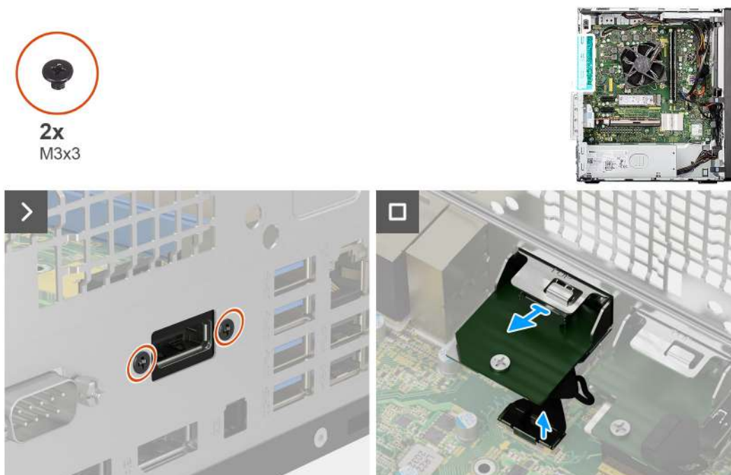
Obrázek 78. Demontáž volitelného modulu DisplayPort
