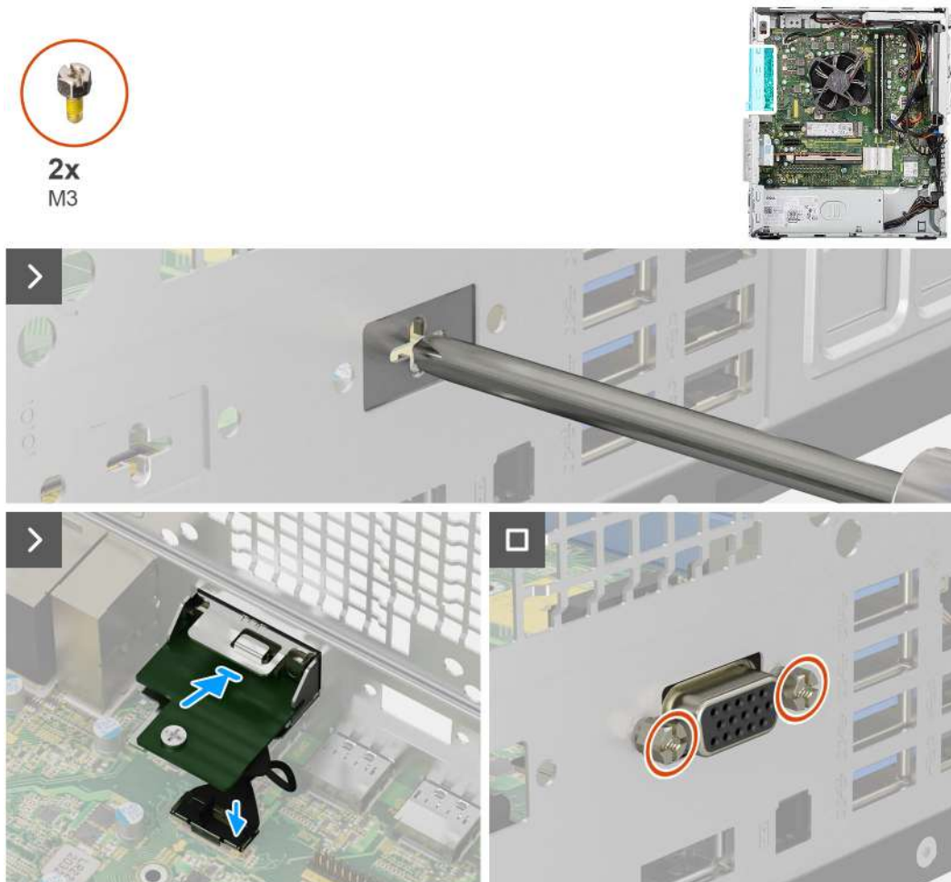
Obrázek 81. Montáž volitelného modulu VGA
