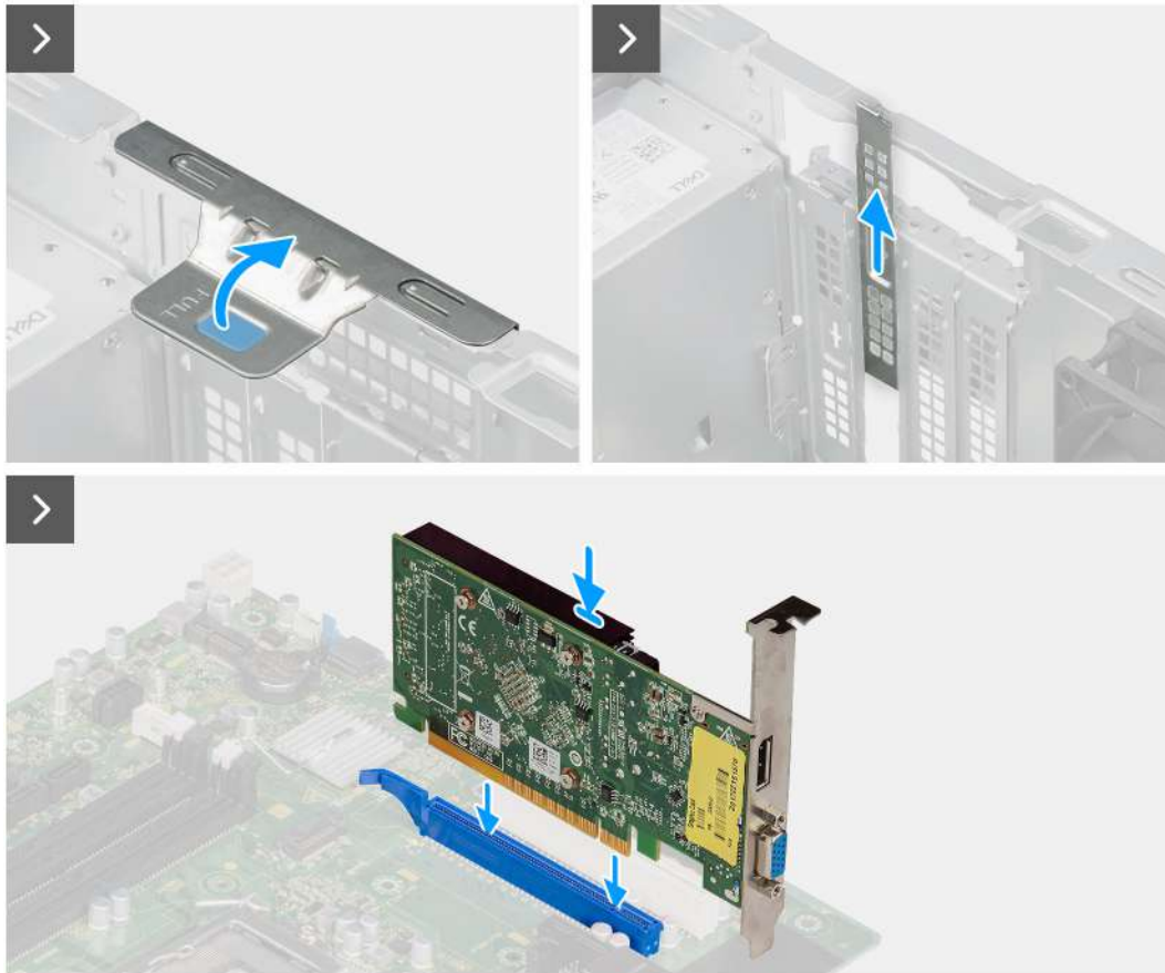
Obrázek 45. Montáž karty sériového/paralelního portu
