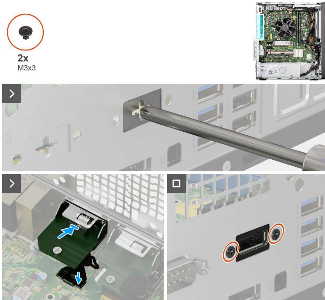
Obrázek 79. Instalace volitelného modulu DisplayPort
