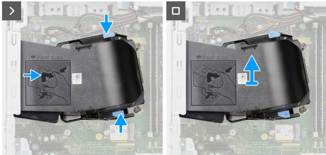
Obrázek 60. Demontáž vedení ventilátoru
