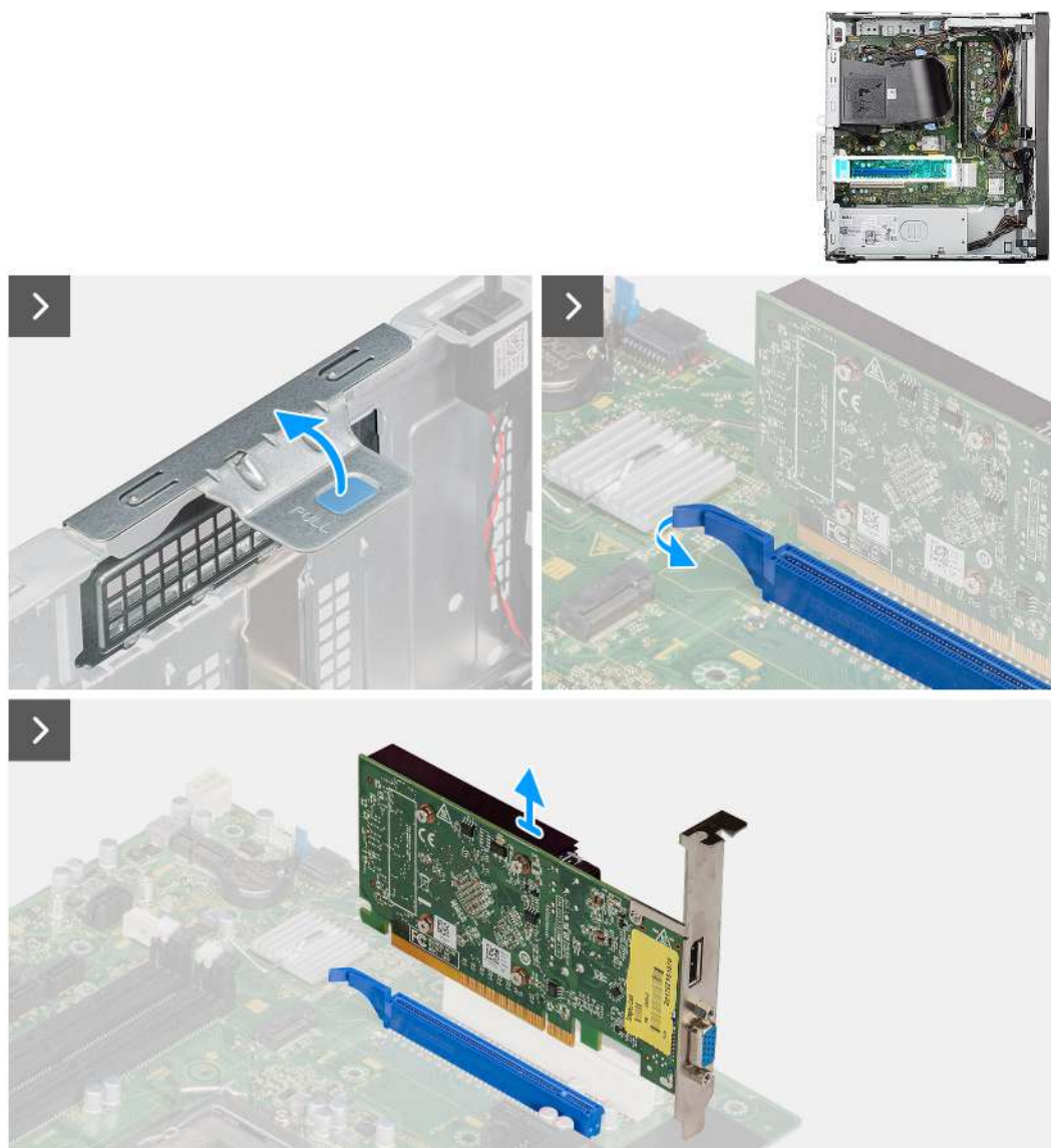
Obrázek 43. Demontáž karty sériového/paralelního portu
