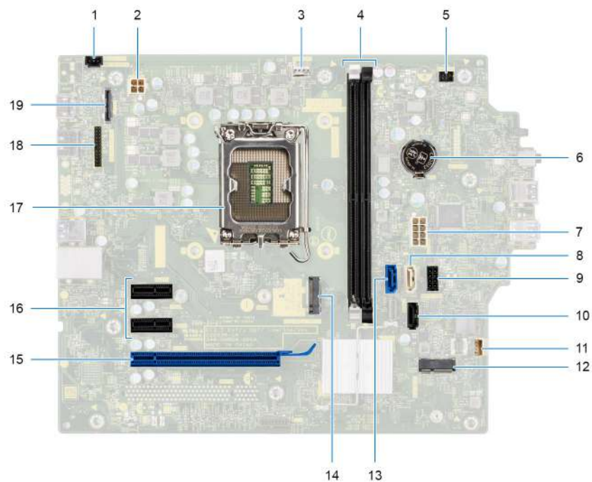
Obrázek 87. Konektory základní desky
