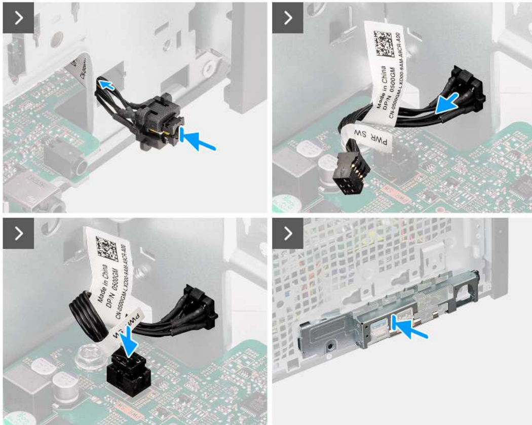
Obrázek 50. Montáž vypínače
