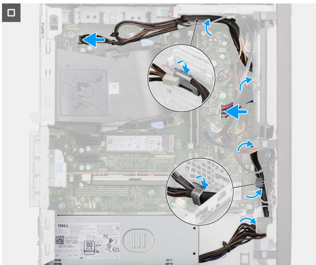
Obrázek 67. Montáž napájecí jednotky
