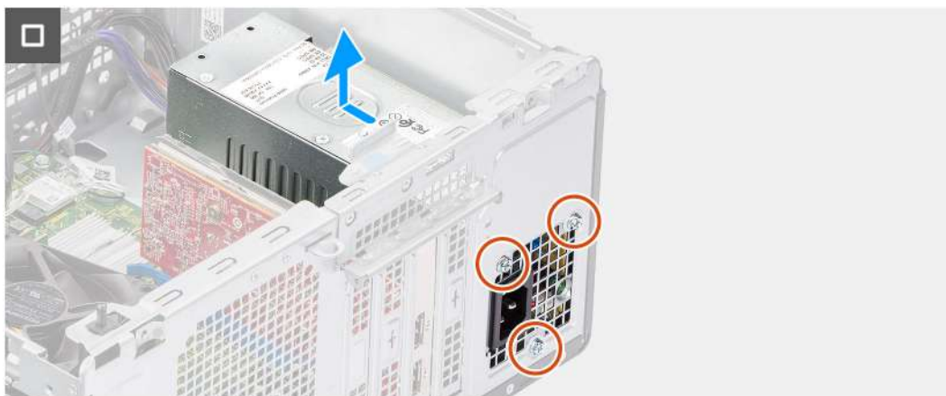
Obrázek 65. Demontáž napájecí jednotky
