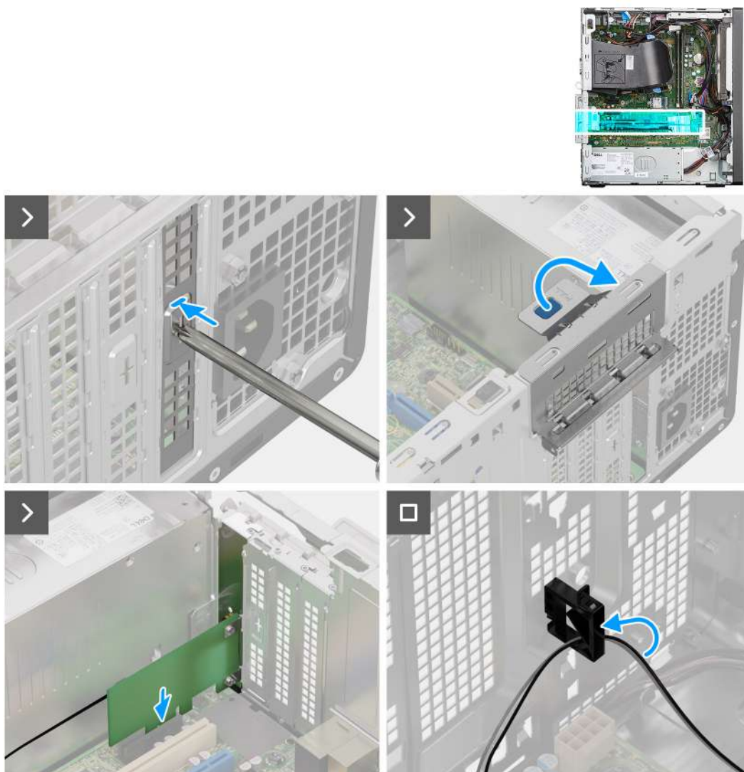
Obrázek 58. Montáž modulu externí antény SMA
