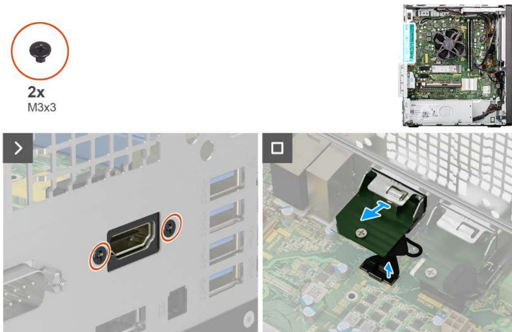
Obrázek 76. Demontáž volitelného modulu HDMI
