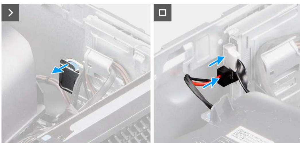
Obrázek 40. Montáž tenké optické jednotky
