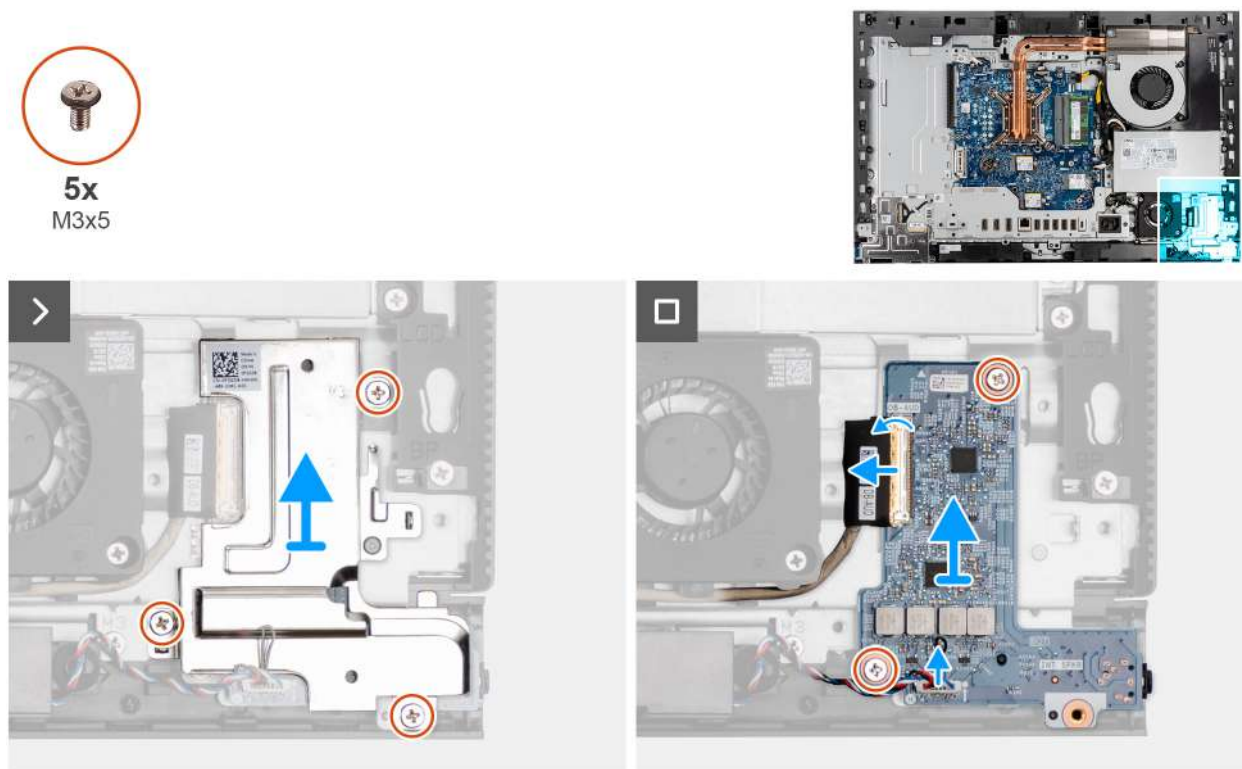
Obrázek 61. Demontáž zvukové karty
