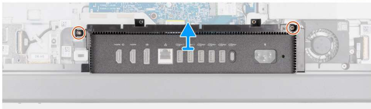
Obrázek 33. Demontáž krytu I/O
