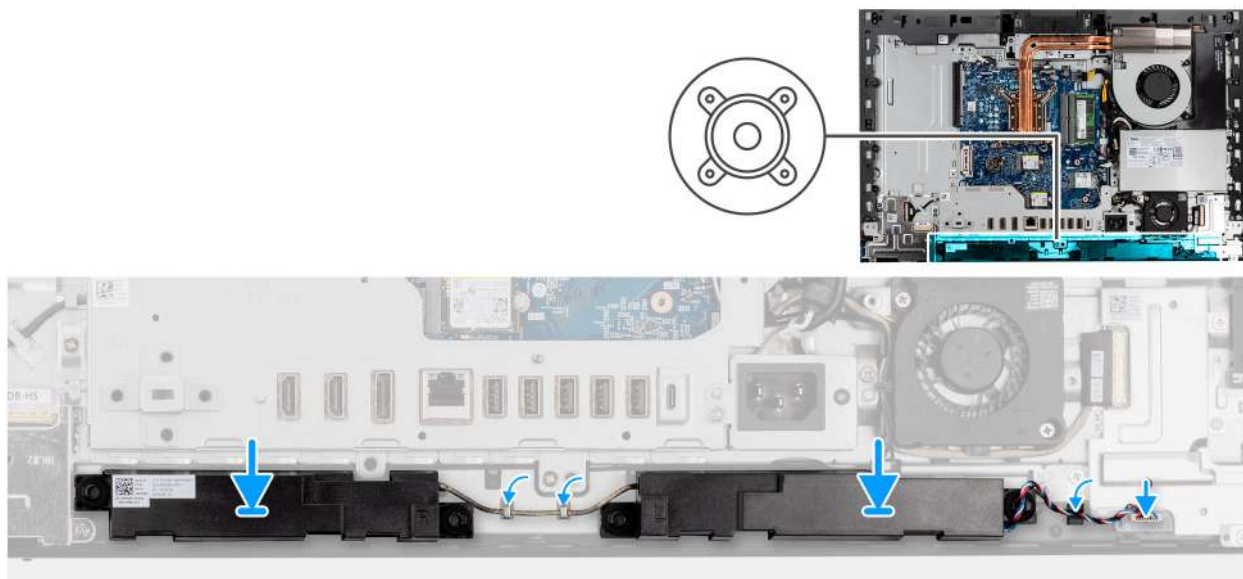
Obrázek 48. Montáž reproduktorů
