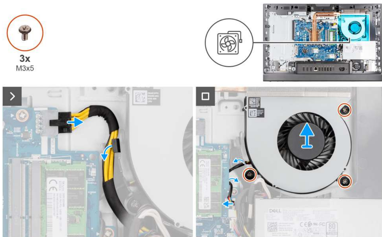
Obrázek 39. Demontáž ventilátoru
