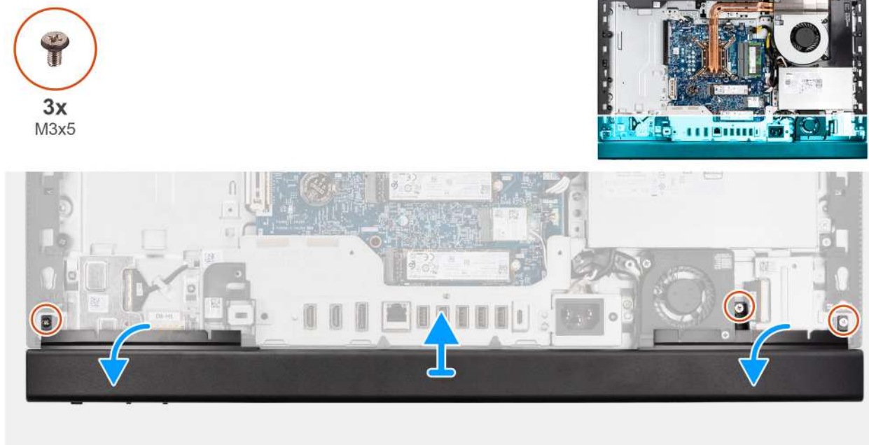
Obrázek 35. Sejmutí spodního krytu
