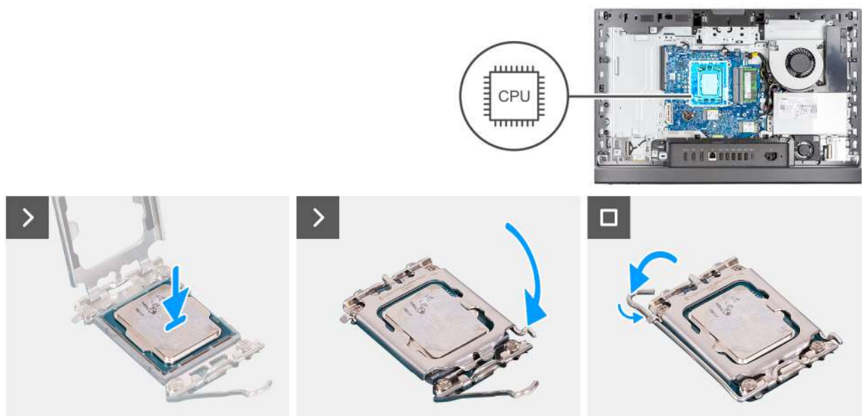
Obrázek 52. Montáž procesoru
