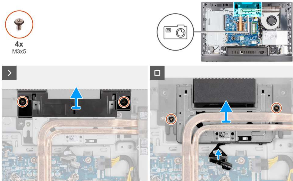
Obrázek 37. Demontáž sestavy zasouvací kamery
