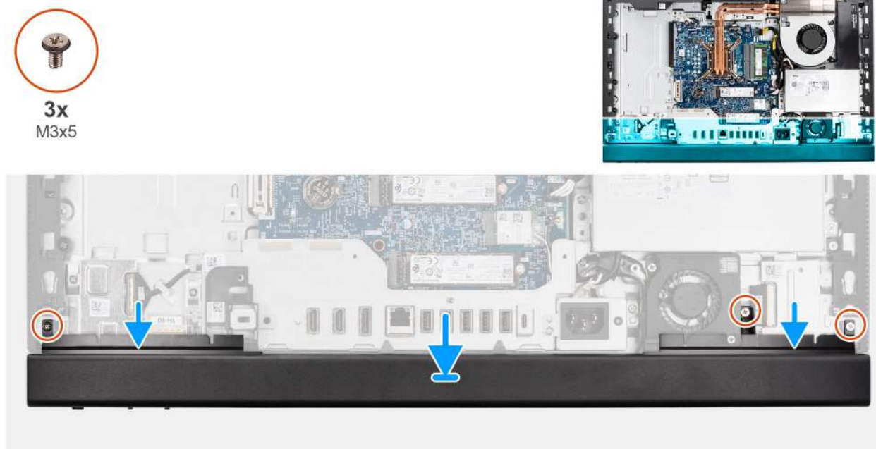
Obrázek 36. Montáž spodního krytu
