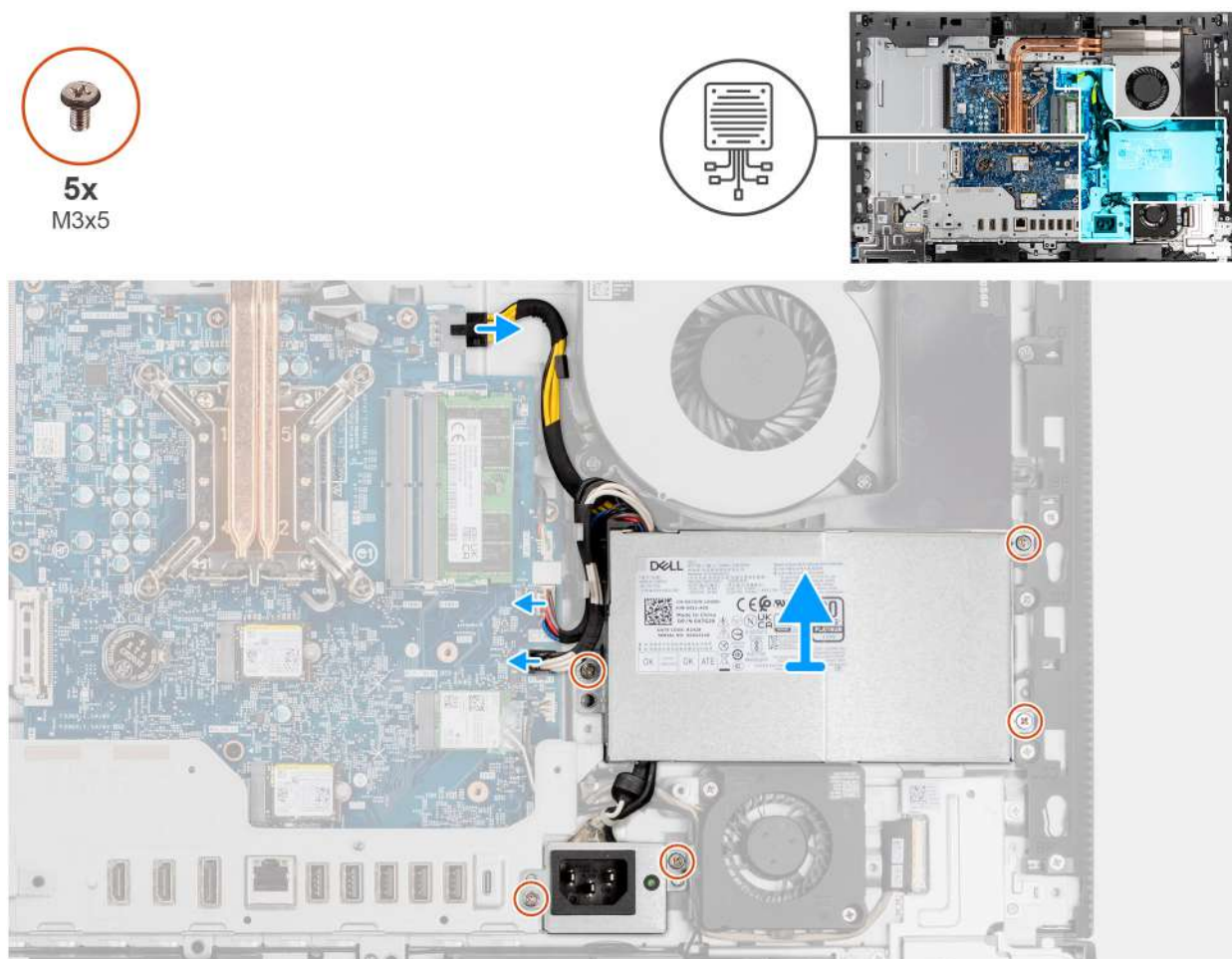
Obrázek 41. Demontáž napájecího zdroje
