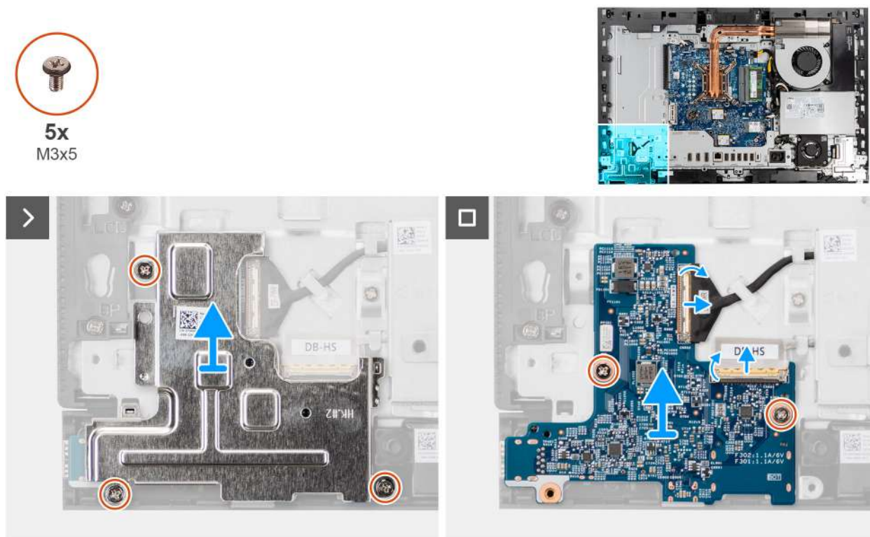
Obrázek 59. Demontáž desky vypínače a I/O
