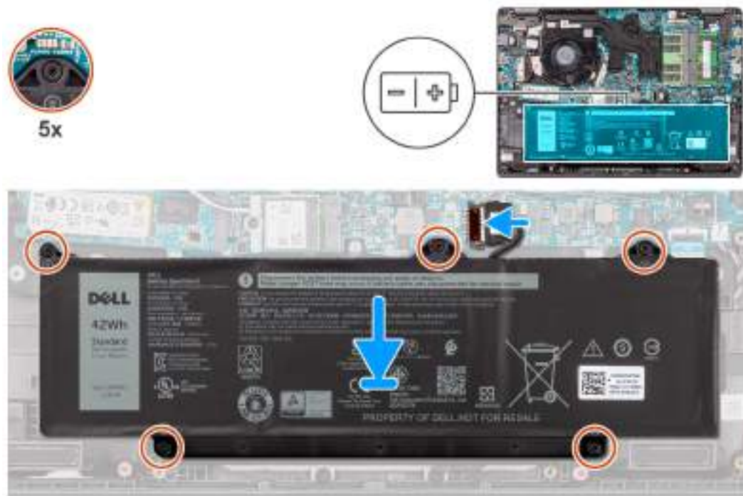
Obrázek 24. Vložení baterie
