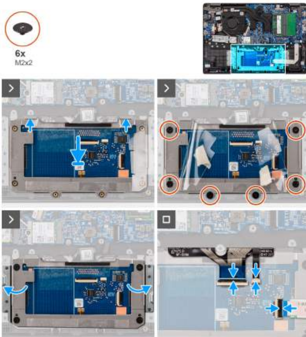
Obrázek 36. Montáž dotykové podložky
