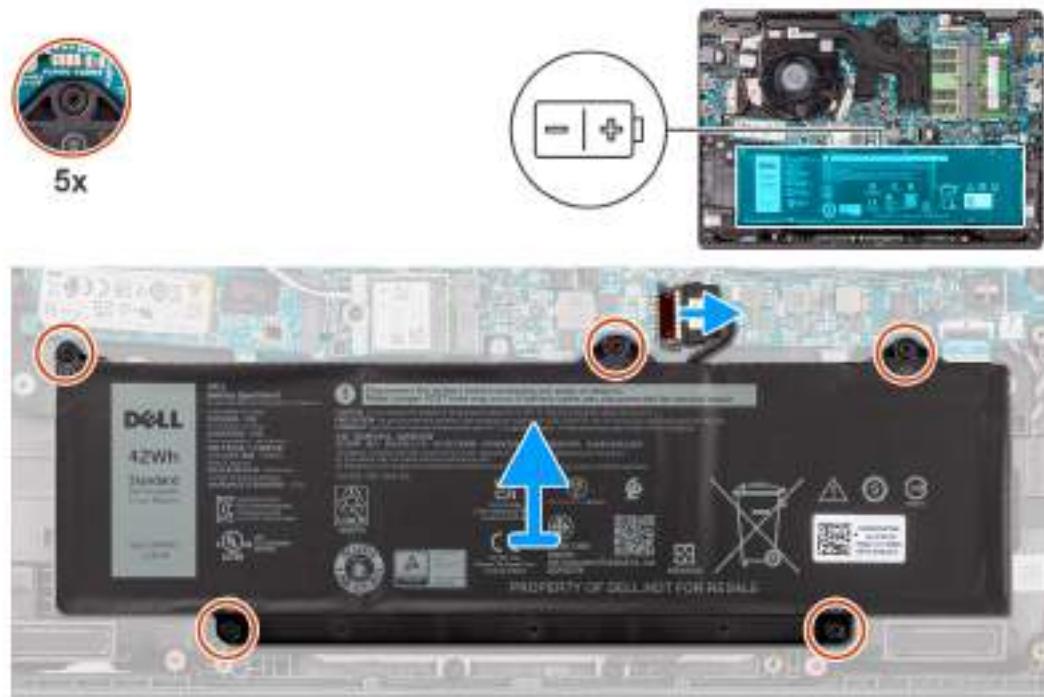
Obrázek 23. Vyjmutí baterie
