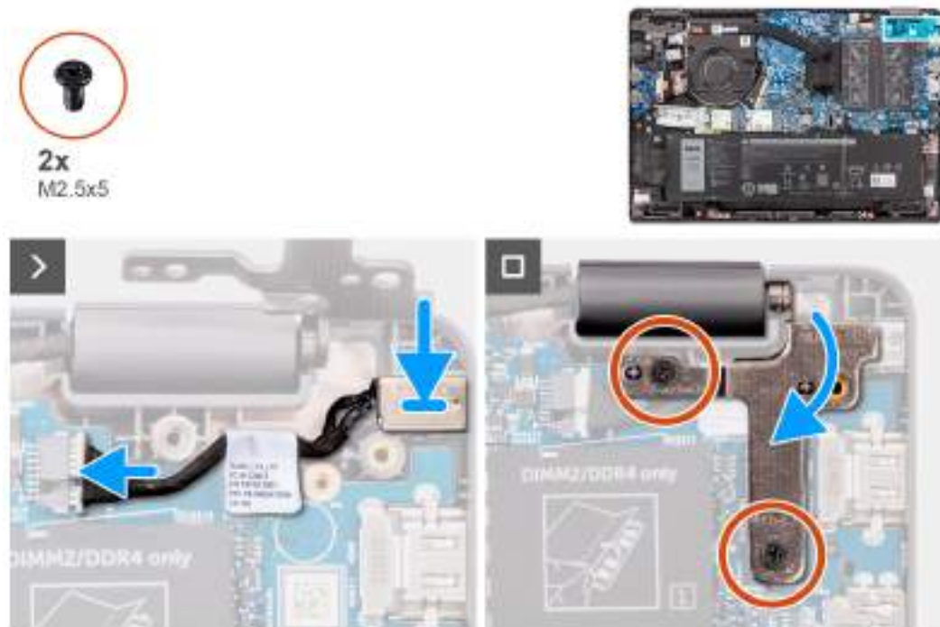
Obrázek 28. Montáž portu napájecího adaptéru
