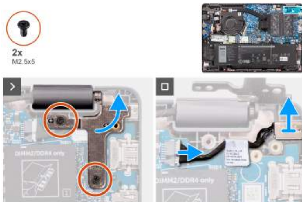
Obrázek 27. Demontáž portu napájecího adaptéru
