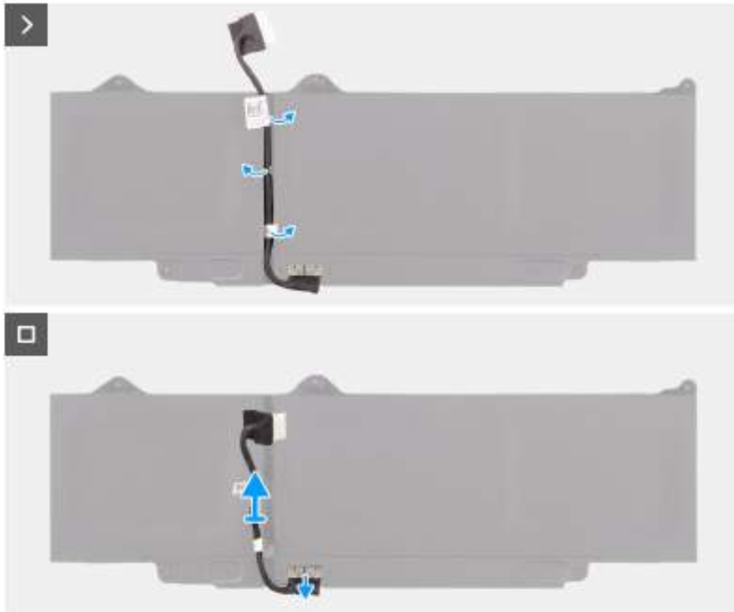
Obrázek 25. Demontáž kabelu baterie
