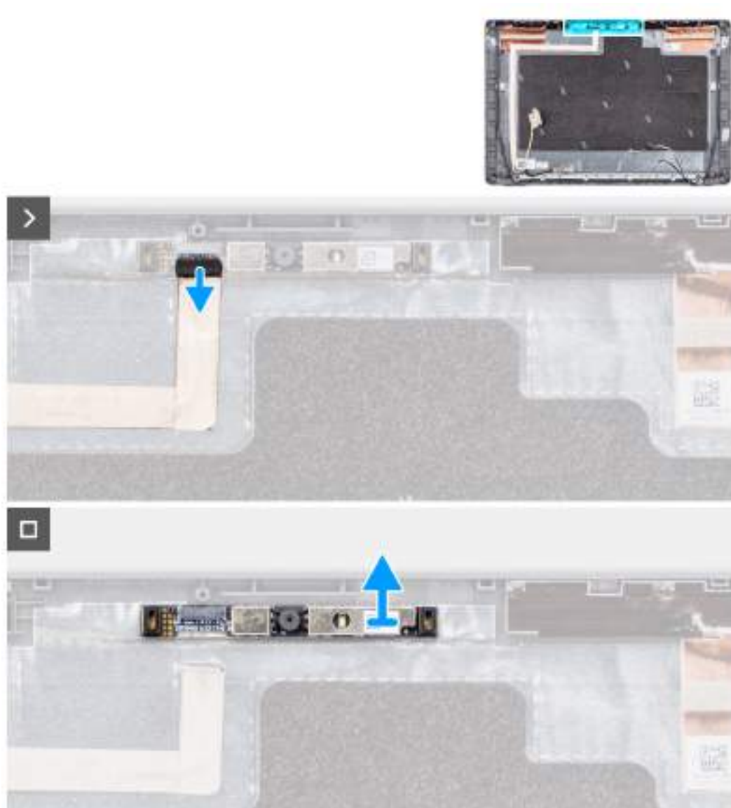
Obrázek 64. Demontáž kamery
