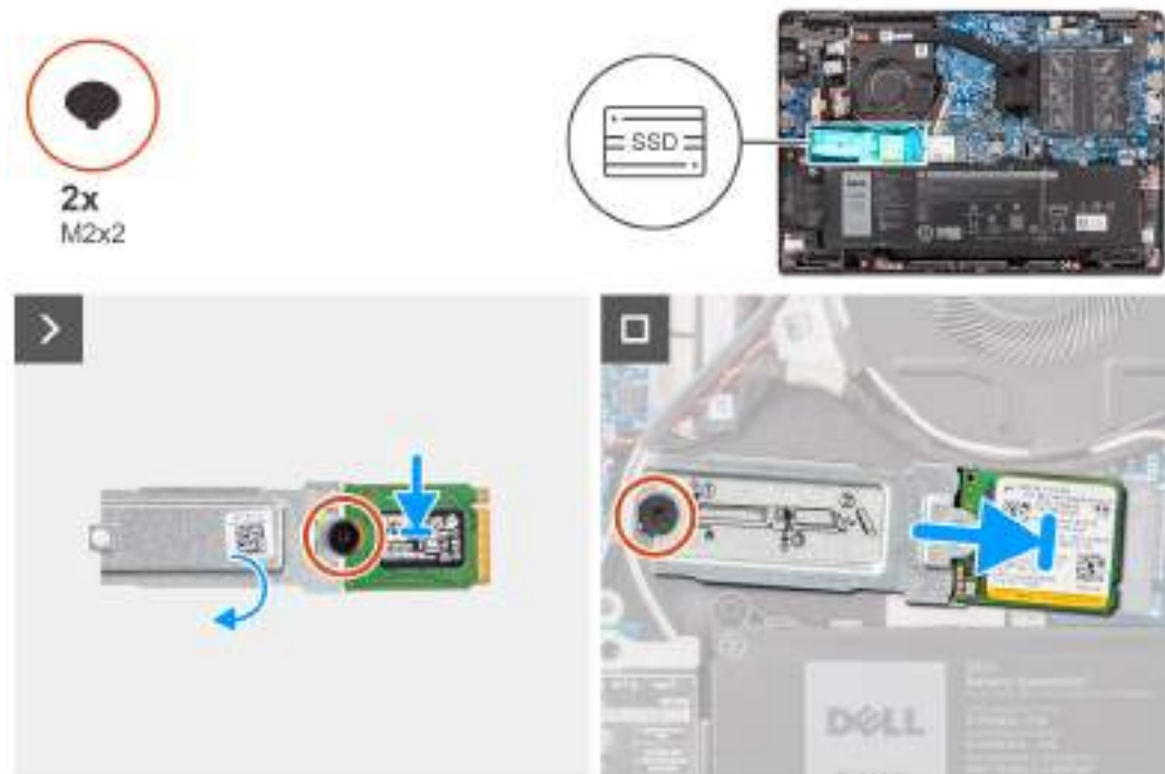
Obrázek 20. Montáž disku SSD M.2 2230
