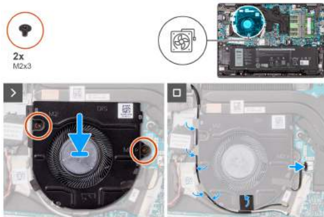
Obrázek 34. Montáž ventilátoru
