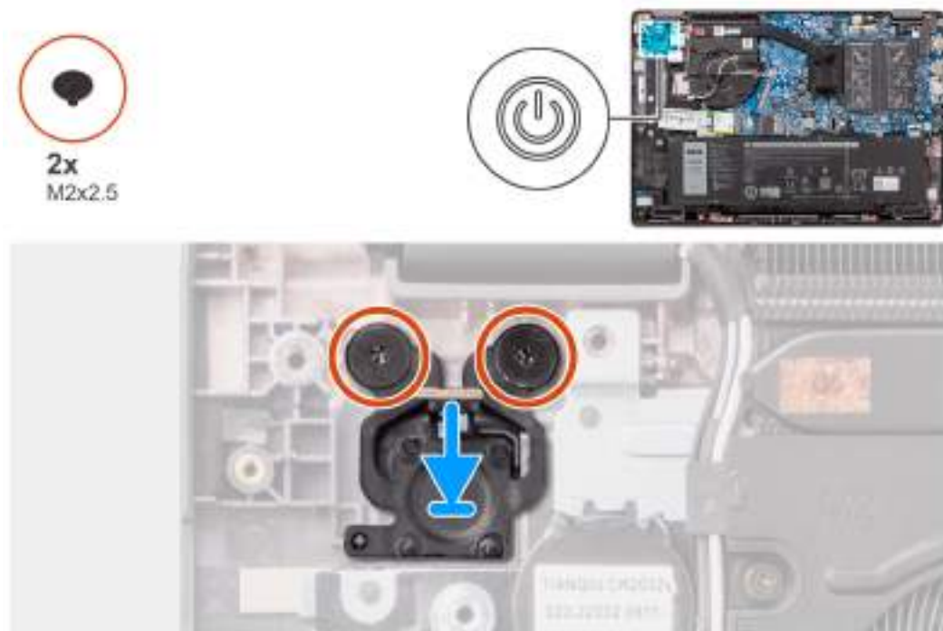
Obrázek 40. Montáž vypínače
