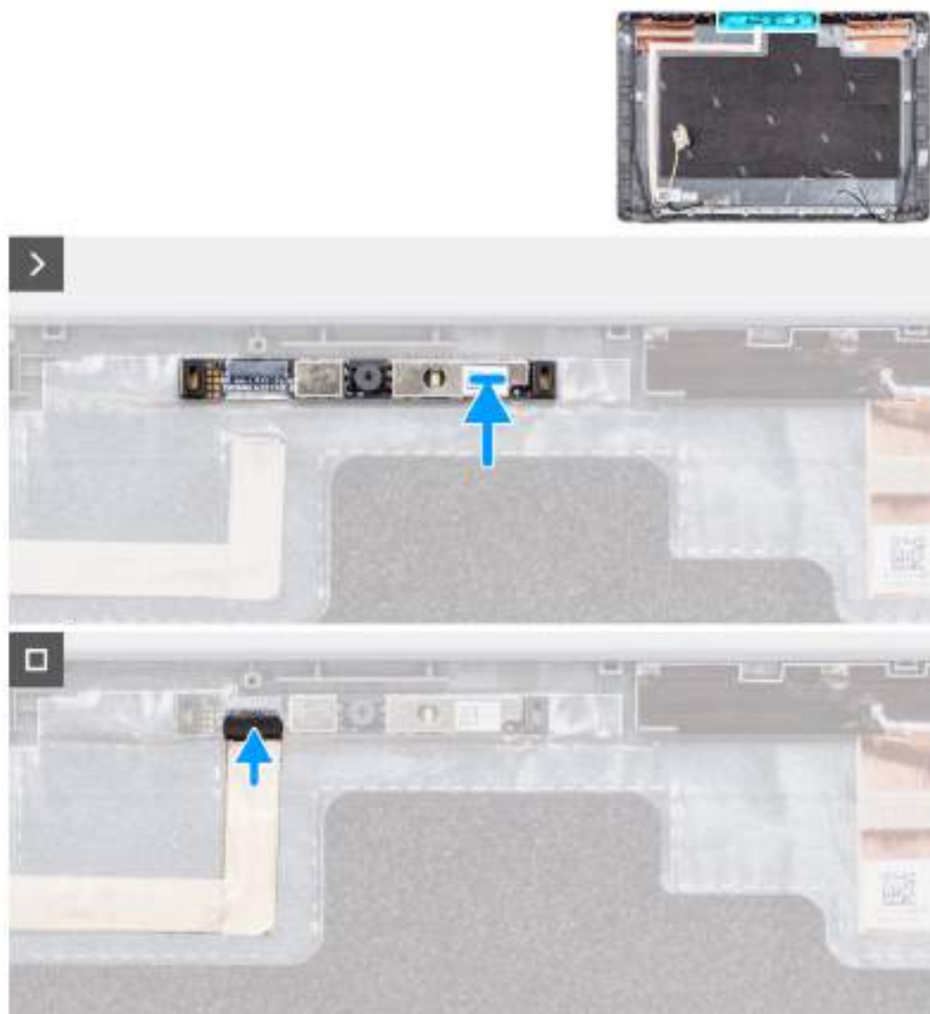
Obrázek 65. Montáž kamery
