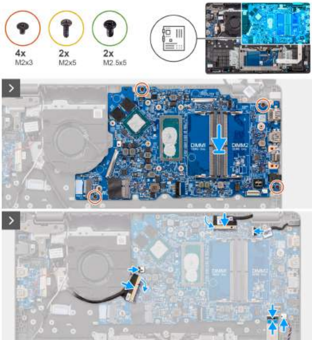
Obrázek 43. Montáž základní desky
