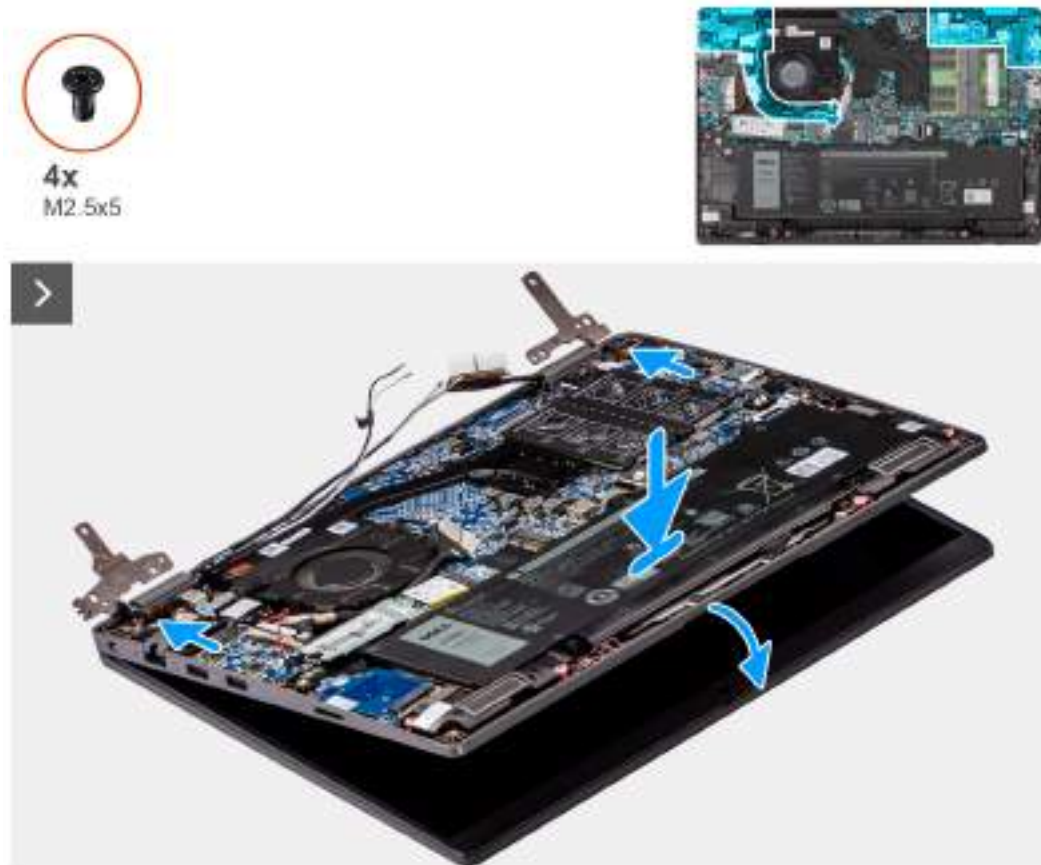
Obrázek 50. Montáž sestavy displeje
