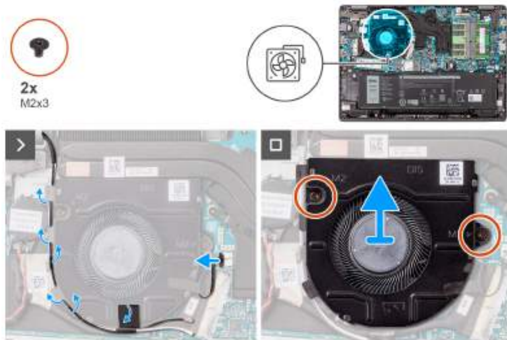
Obrázek 33. Demontáž ventilátoru
