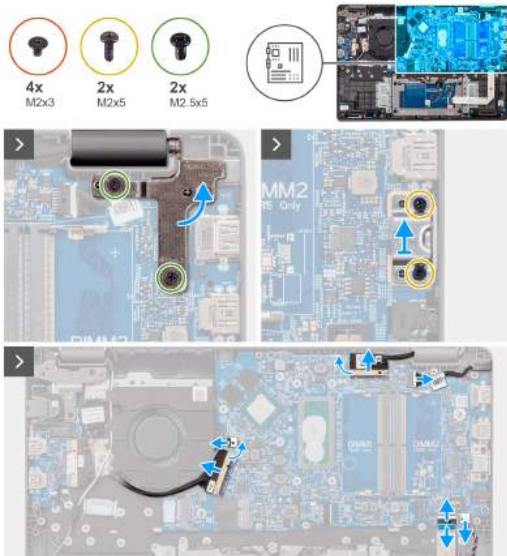
Obrázek 42. Demontáž základní desky
