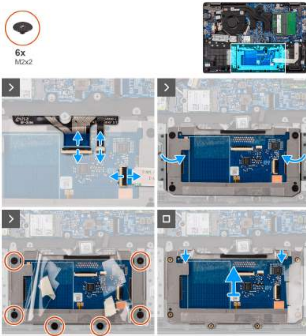
Obrázek 35. Demontáž dotykové podložky
