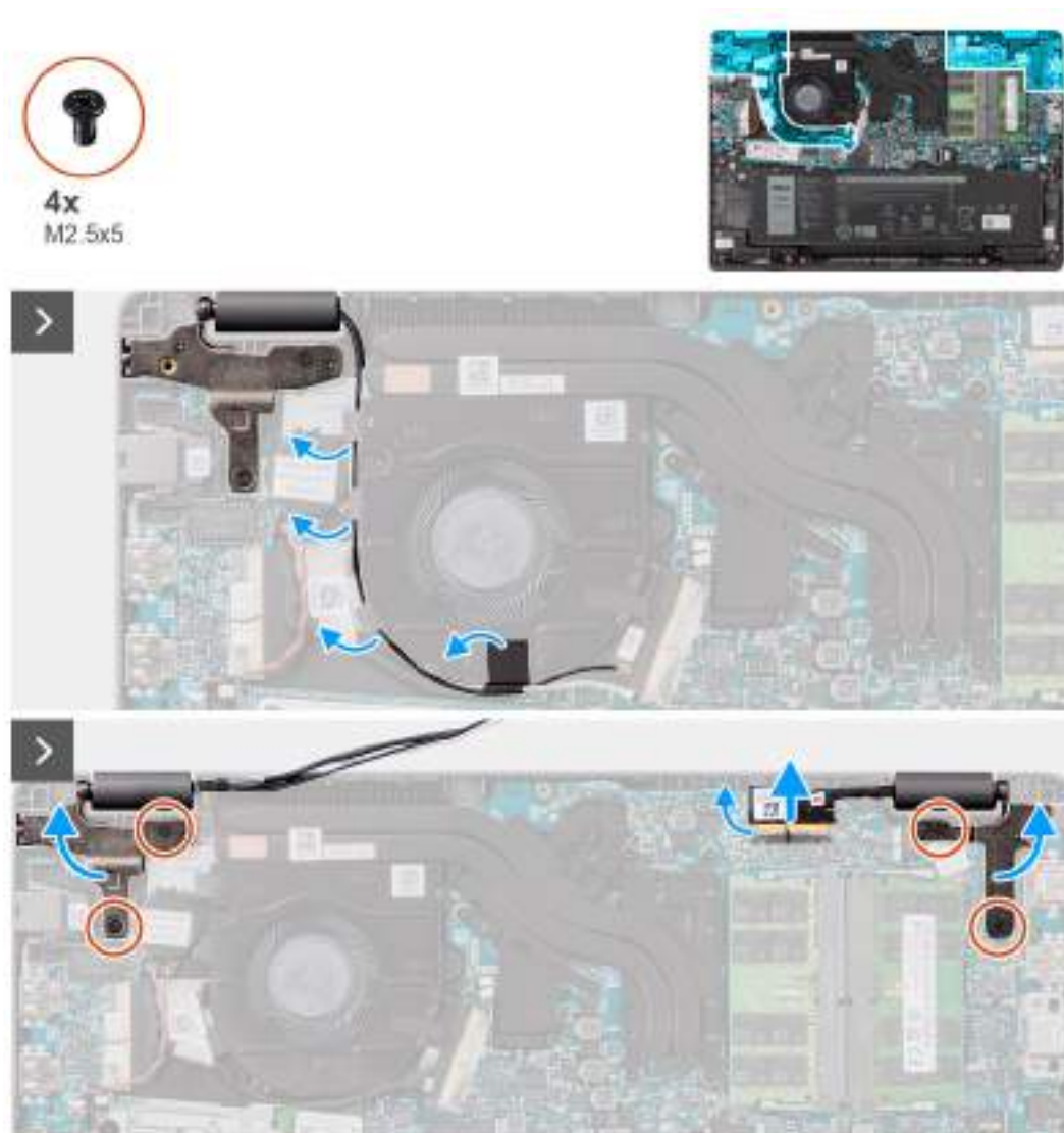
Obrázek 47. Demontáž sestavy displeje
