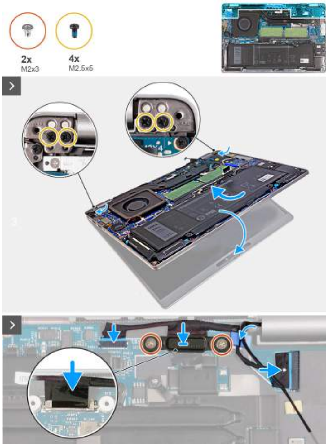
Obrázek 52. Montáž sestavy displeje – u počítačů dodávaných se samostatnou grafickou kartou
