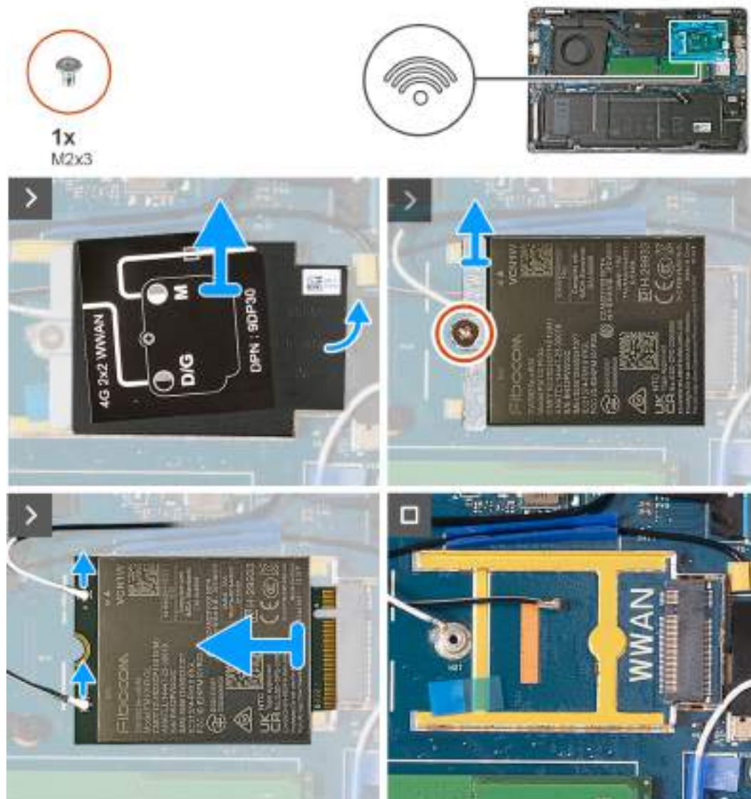
Obrázek 20. Demontáž karty WWAN – pro počítače dodávané s kartou 4G
