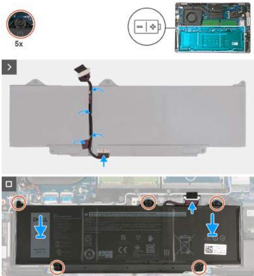
Obrázek 27. Vložení baterie
