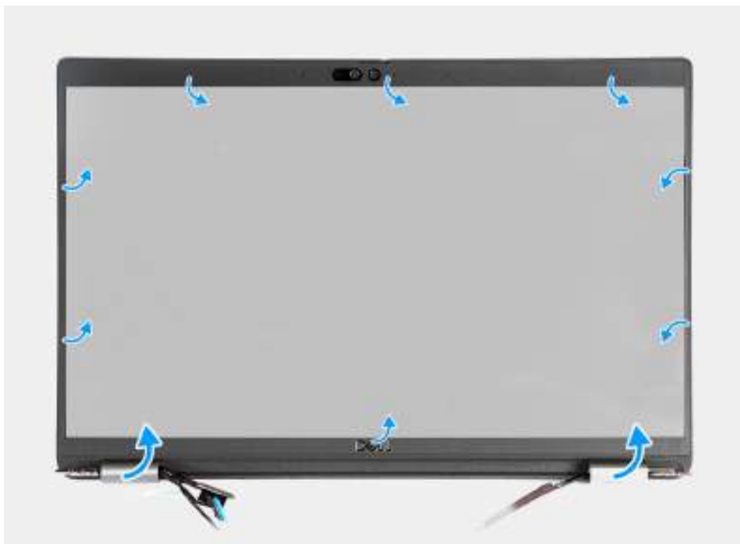
Obrázek 53. Demontáž čelního krytu displeje
