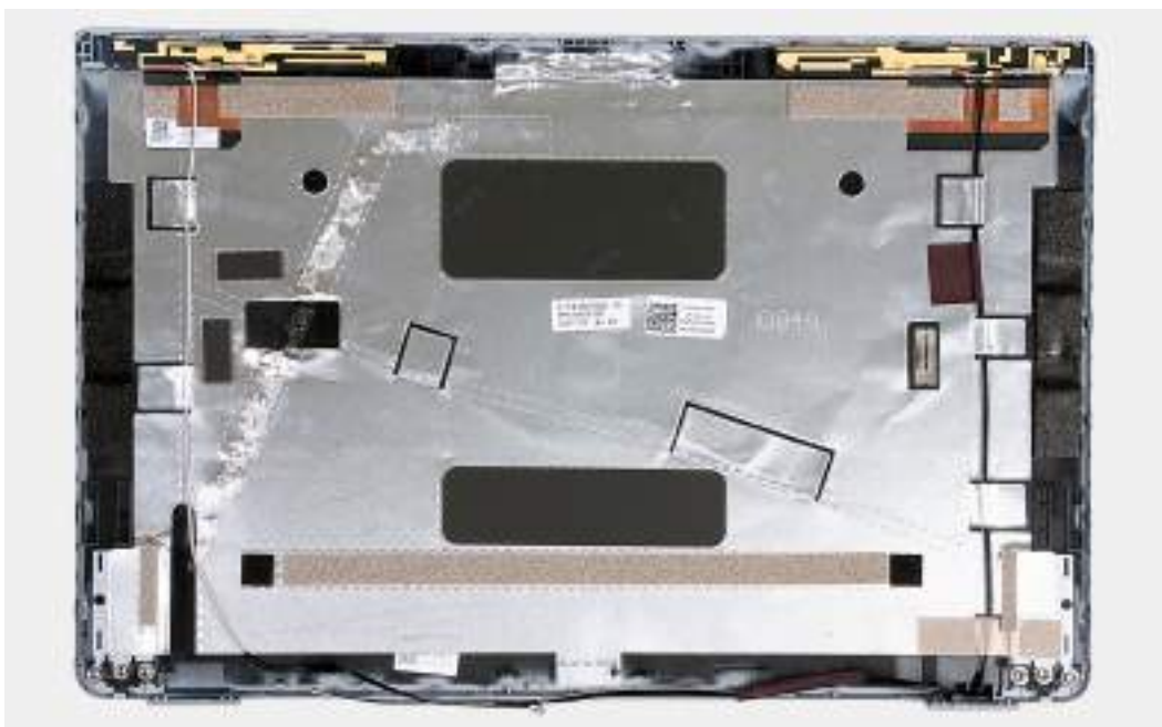
Obrázek 64. Demontáž zadního krytu displeje
