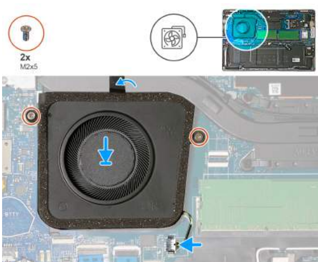
Obrázek 25. Montáž ventilátoru
