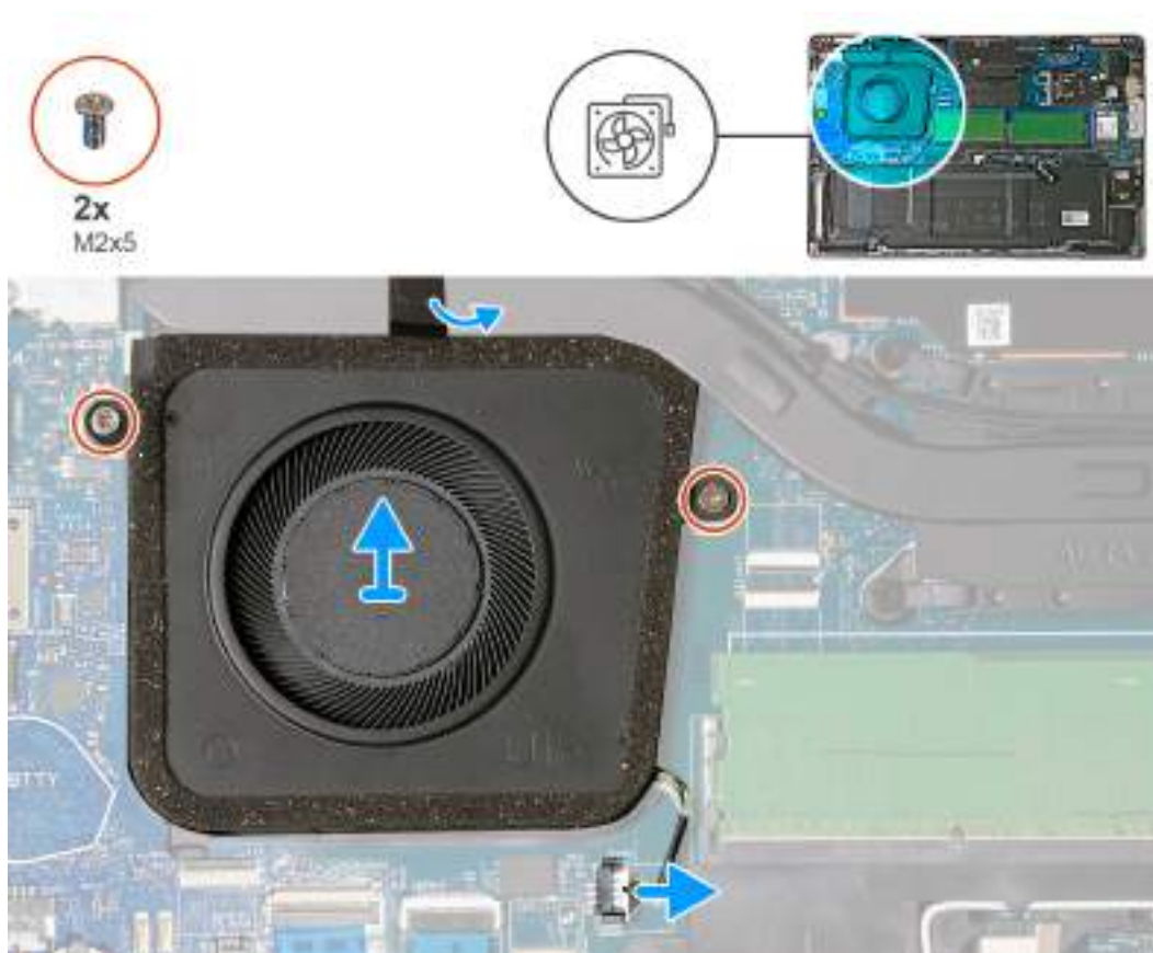
Obrázek 24. Demontáž ventilátoru
