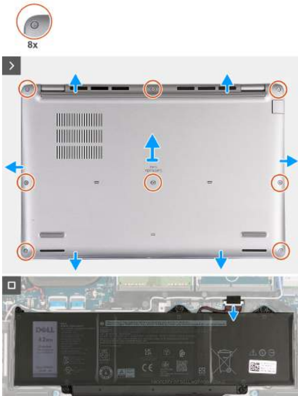
Obrázek 12. Sejmutí spodního krytu
