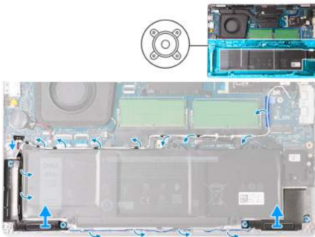
Obrázek 38. Demontáž reproduktorů
