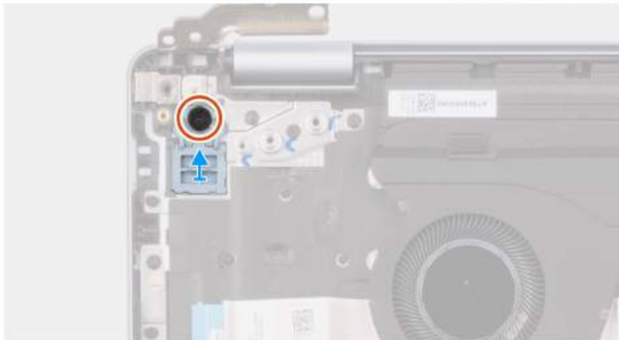
Obrázek 51. Demontáž vypínače
