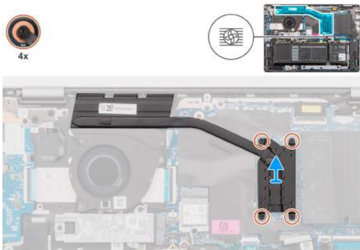
Obrázek 37. Demontáž chladiče – v počítačích dodávaných s integrovanou grafickou kartou
