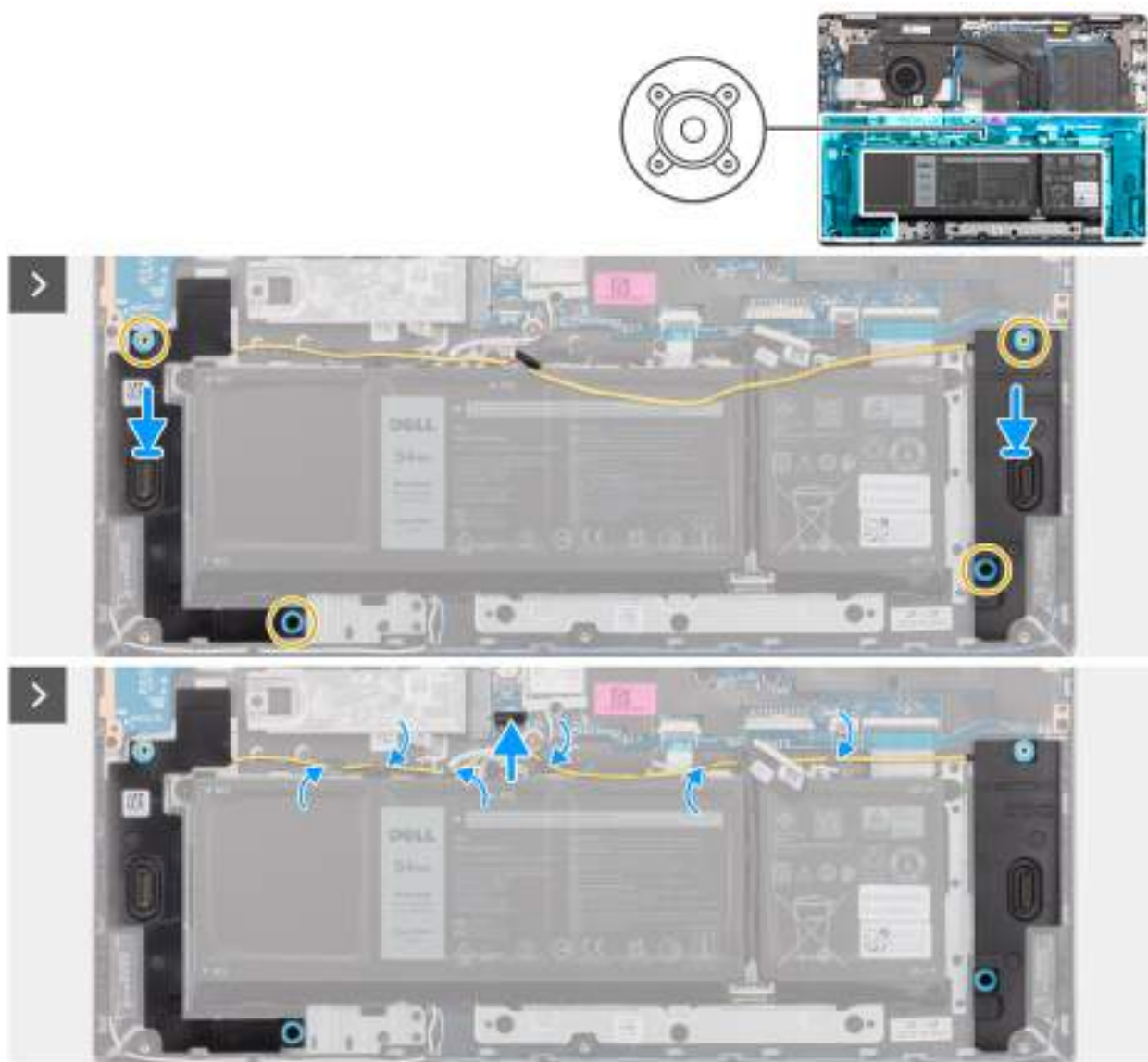
Obrázek 32. Montáž reproduktorů
