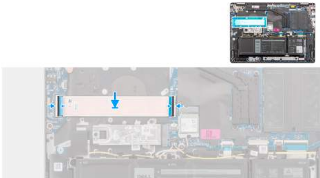
Obrázek 44. Montáž kabelu desky I/O
