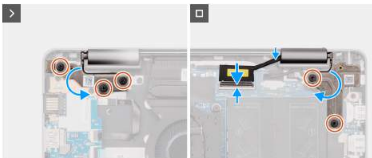
Obrázek 50. Montáž sestavy displeje
