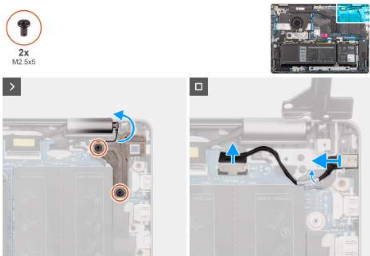
Obrázek 56. Demontáž portu napájecího adaptéru
