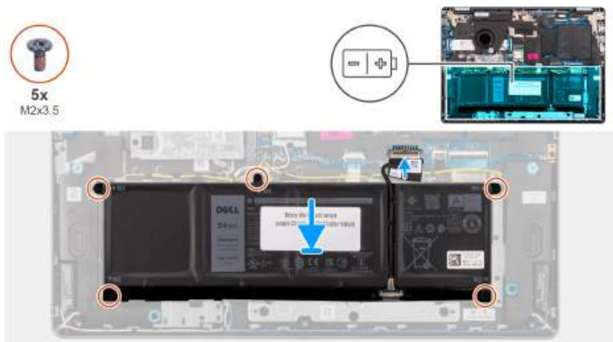
Obrázek 17. Vložení baterie
