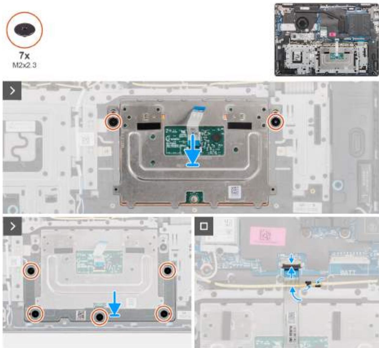
Obrázek 42. Montáž dotykové podložky
