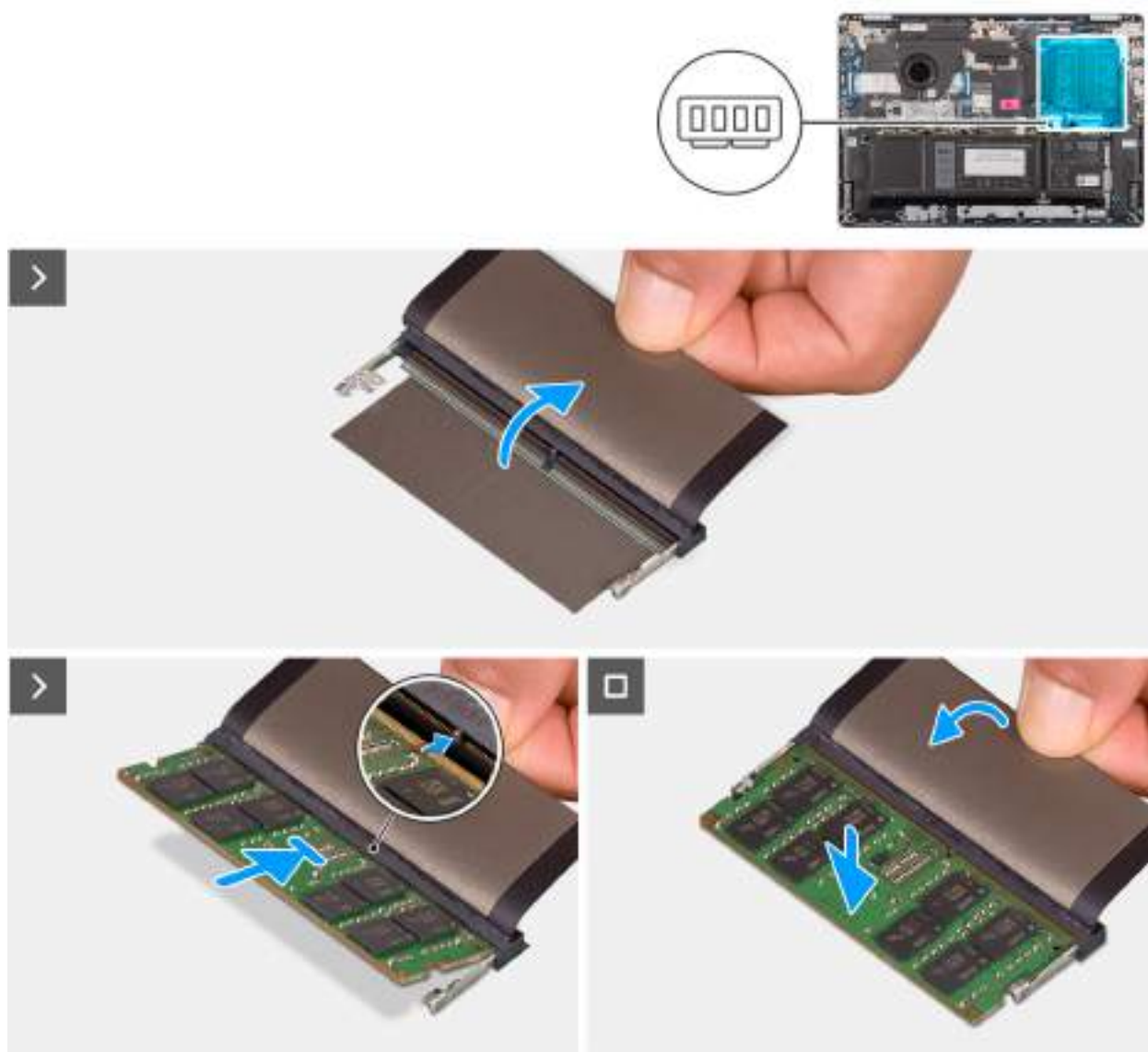
Obrázek 24. Vložení paměťového modulu
