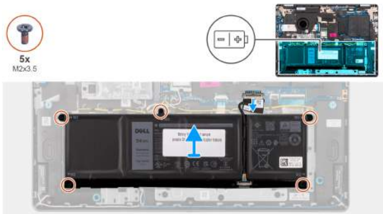
Obrázek 16. Vyjmutí baterie
