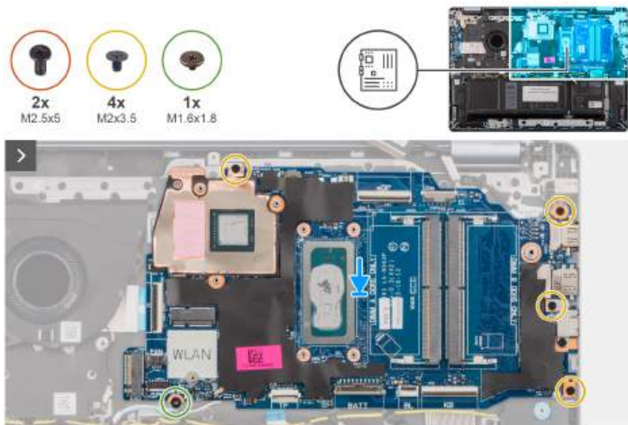
Obrázek 64. Montáž základní desky
