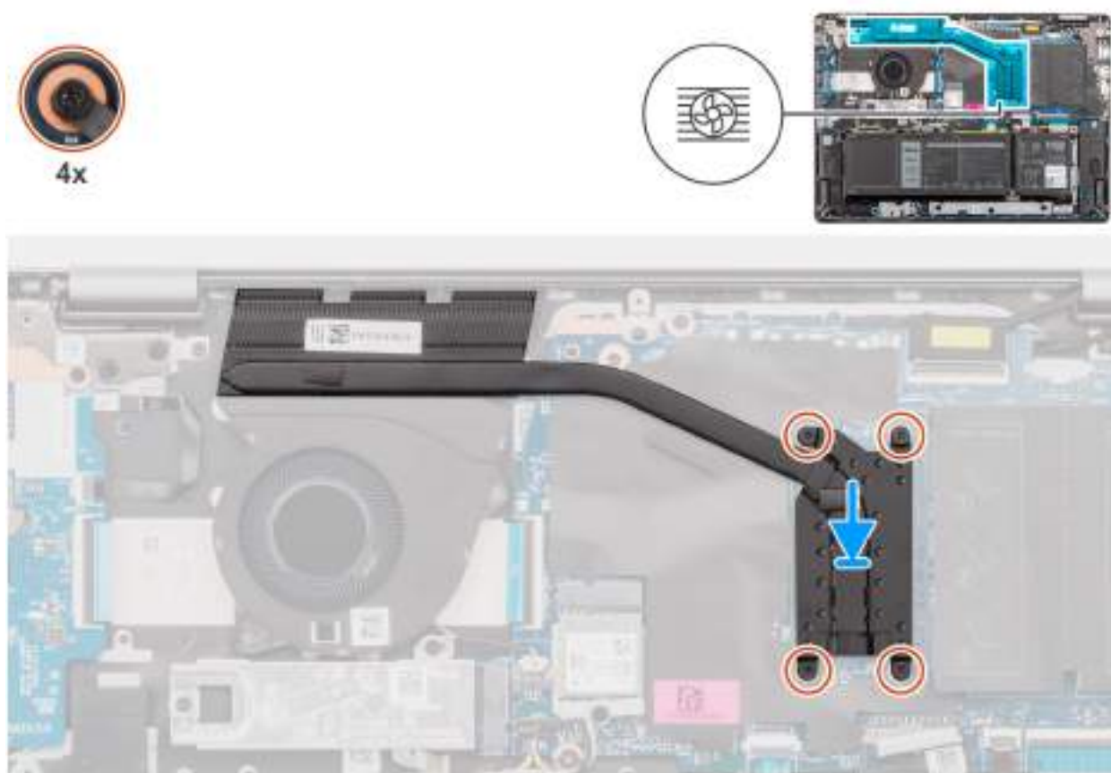
Obrázek 38. Montáž chladiče – v počítačích dodávaných s integrovanou grafickou kartou
