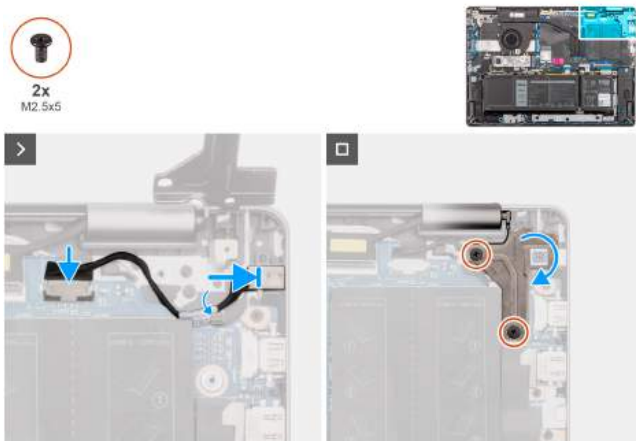
Obrázek 57. Montáž portu napájecího adaptéru
