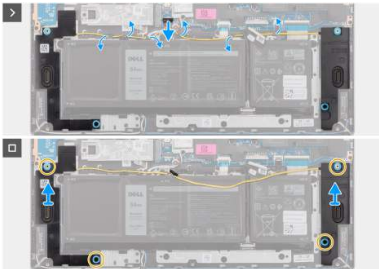
Obrázek 30. Demontáž reproduktorů
