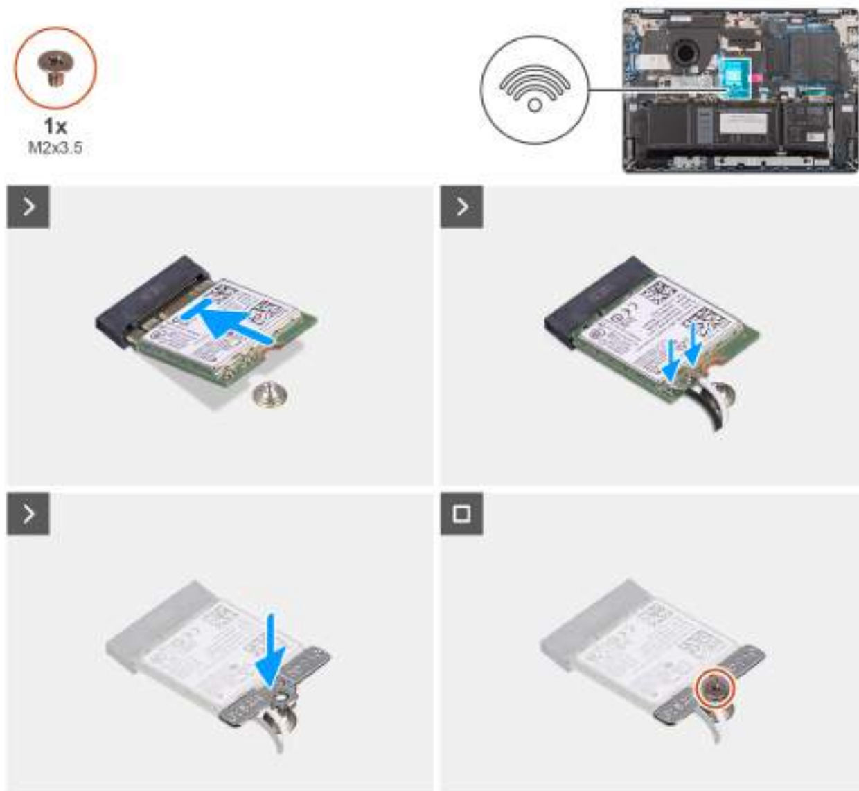
Obrázek 28. Montáž bezdrátové karty
