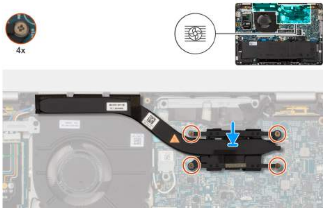
Obrázek 31. Montáž chladiče (integrovaná grafická karta)
