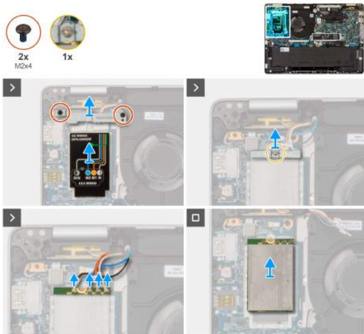
Obrázek 11. Vyjmutí karty 5G WWAN
