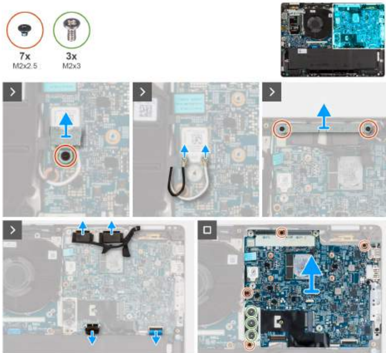
Obrázek 33. Demontáž základní desky
