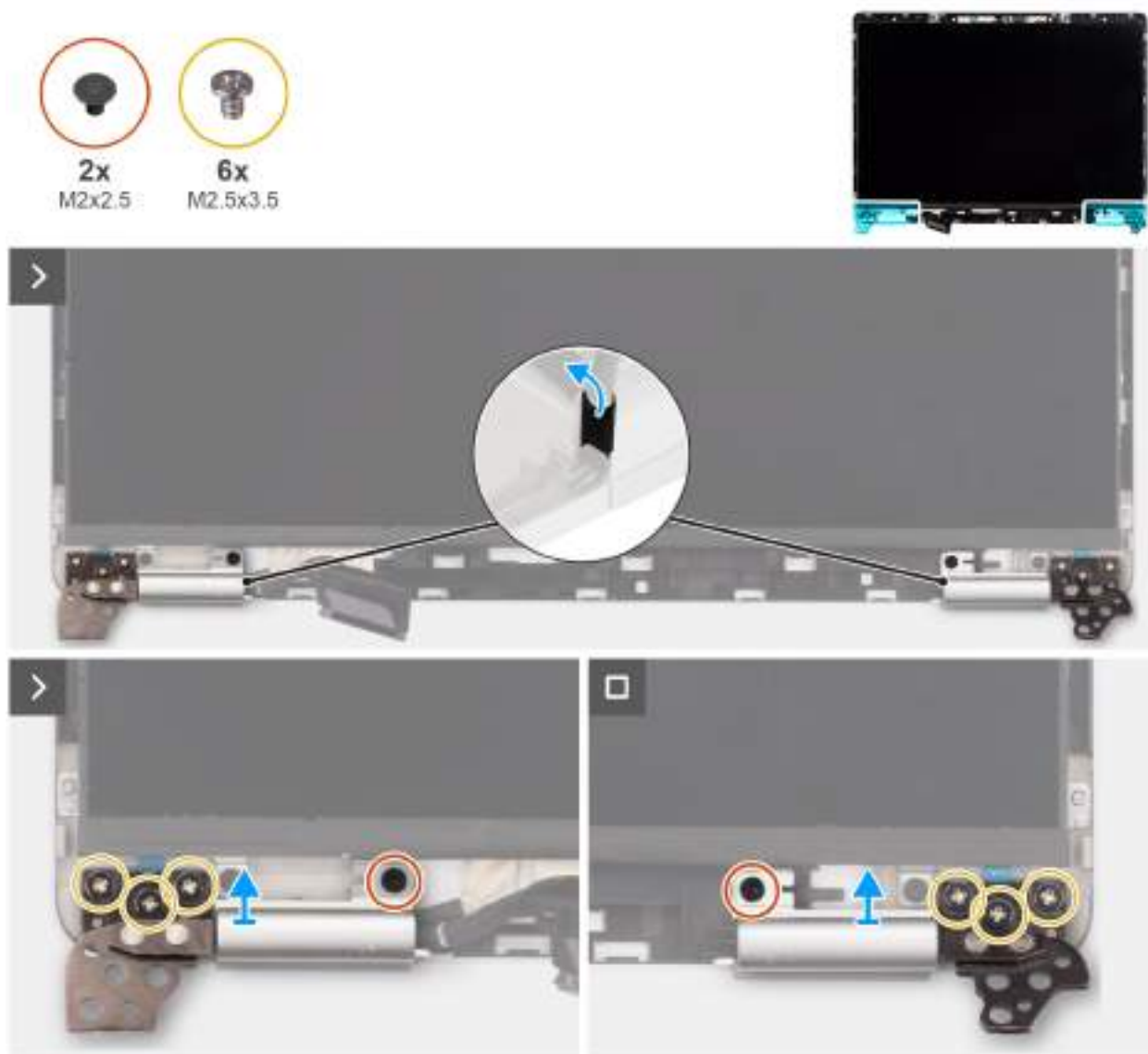
Obrázek 49. Demontáž pantů displeje
