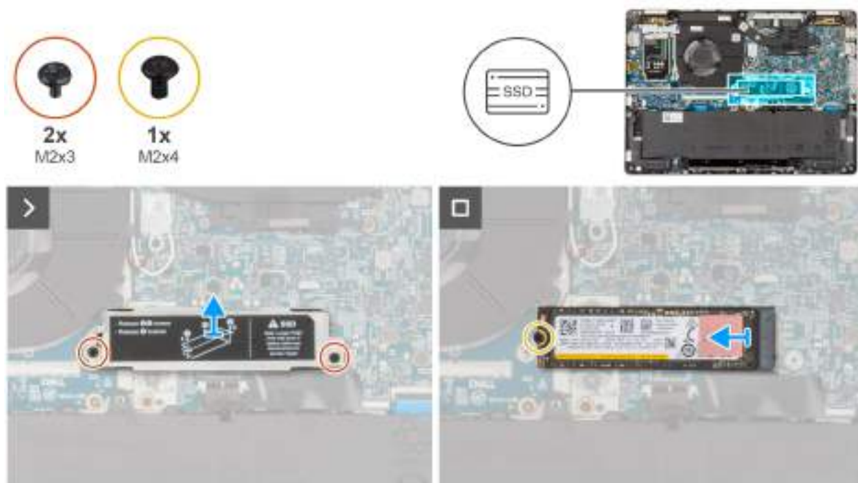
Obrázek 28. Demontáž disku SSD M.2 2280
