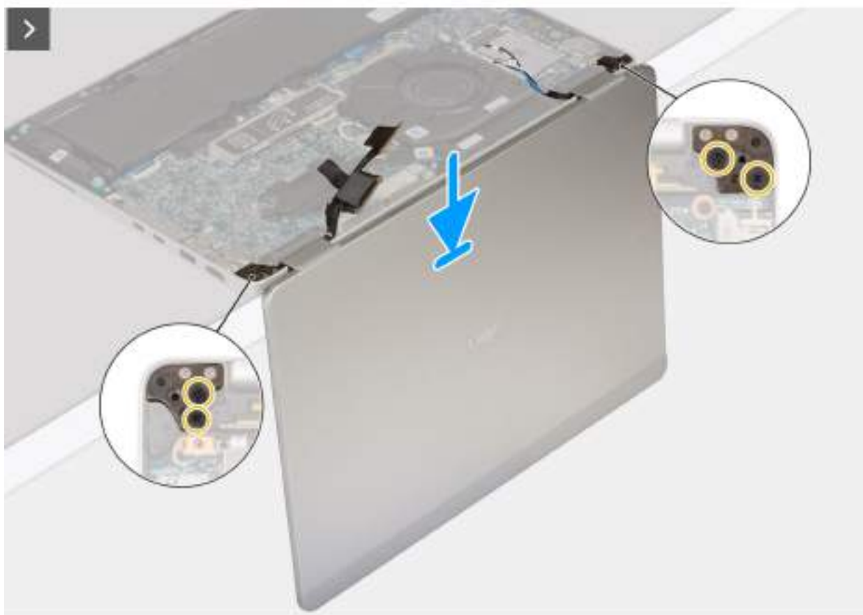
Obrázek 46. Montáž sestavy displeje
