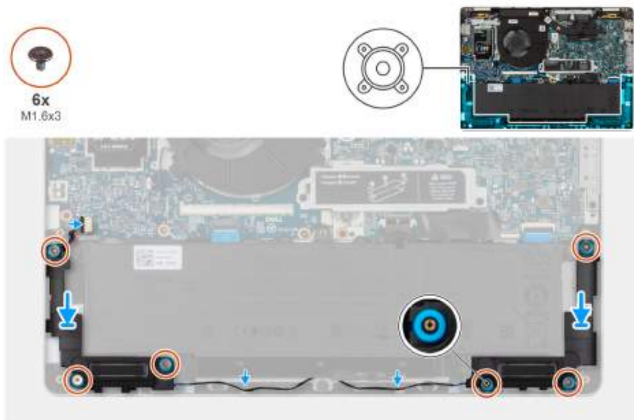
Obrázek 18. Montáž reproduktorů
