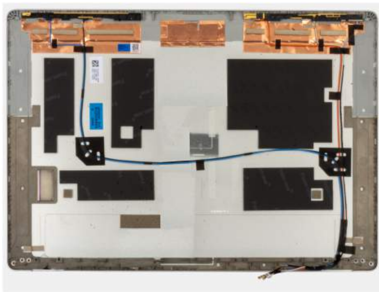
Obrázek 60. Montáž zadního krytu displeje
