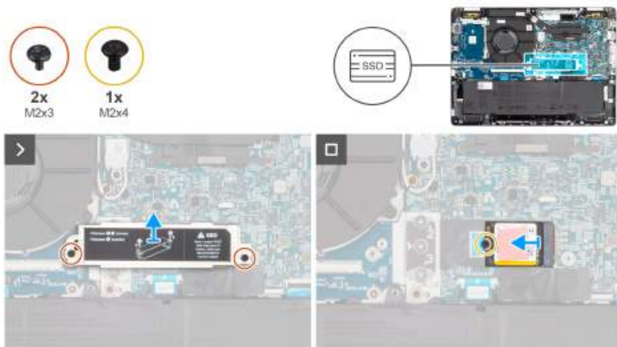
Obrázek 13. Demontáž disku SSD M.2 2230
