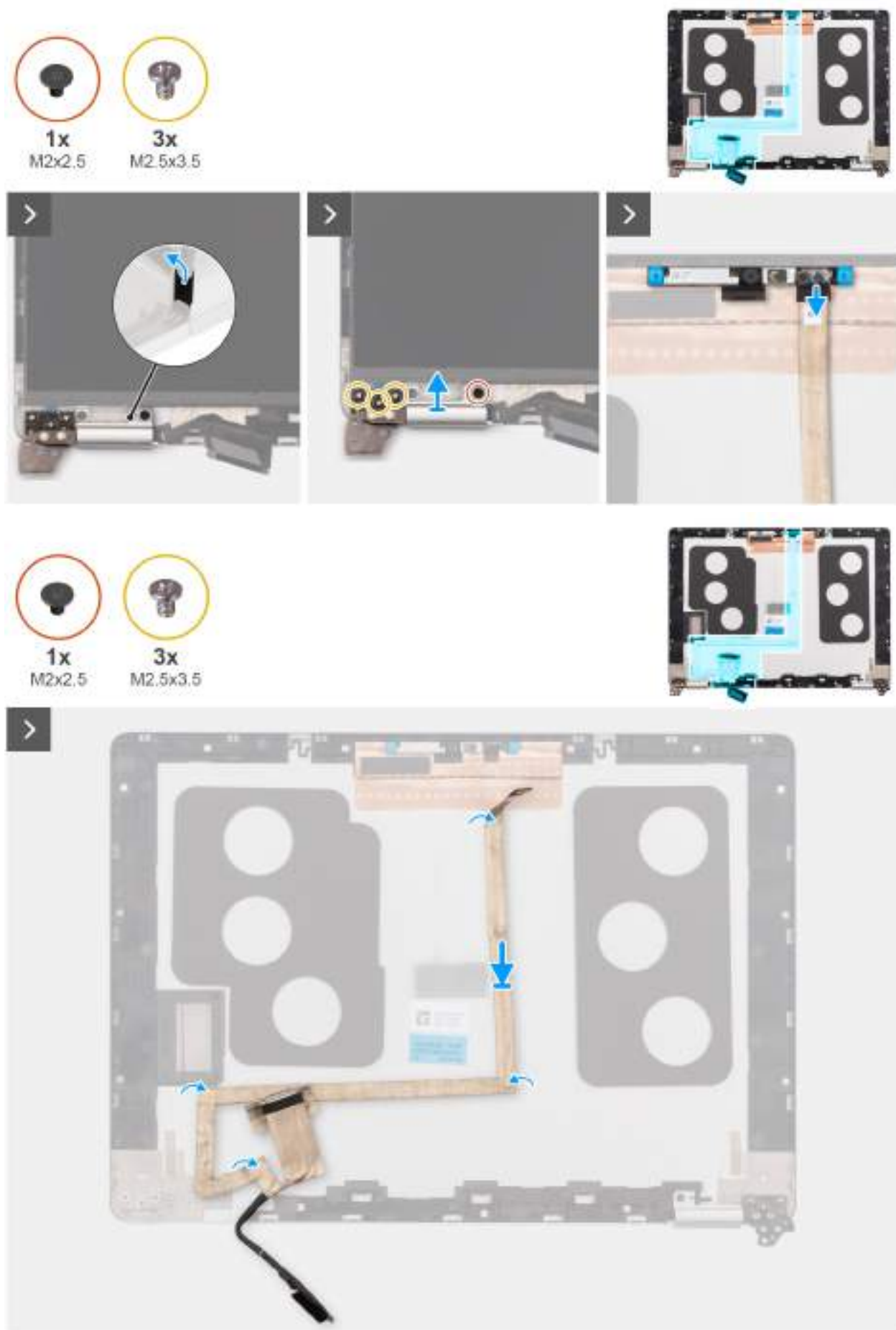
Obrázek 57. Vyjmutí kabelu displeje
