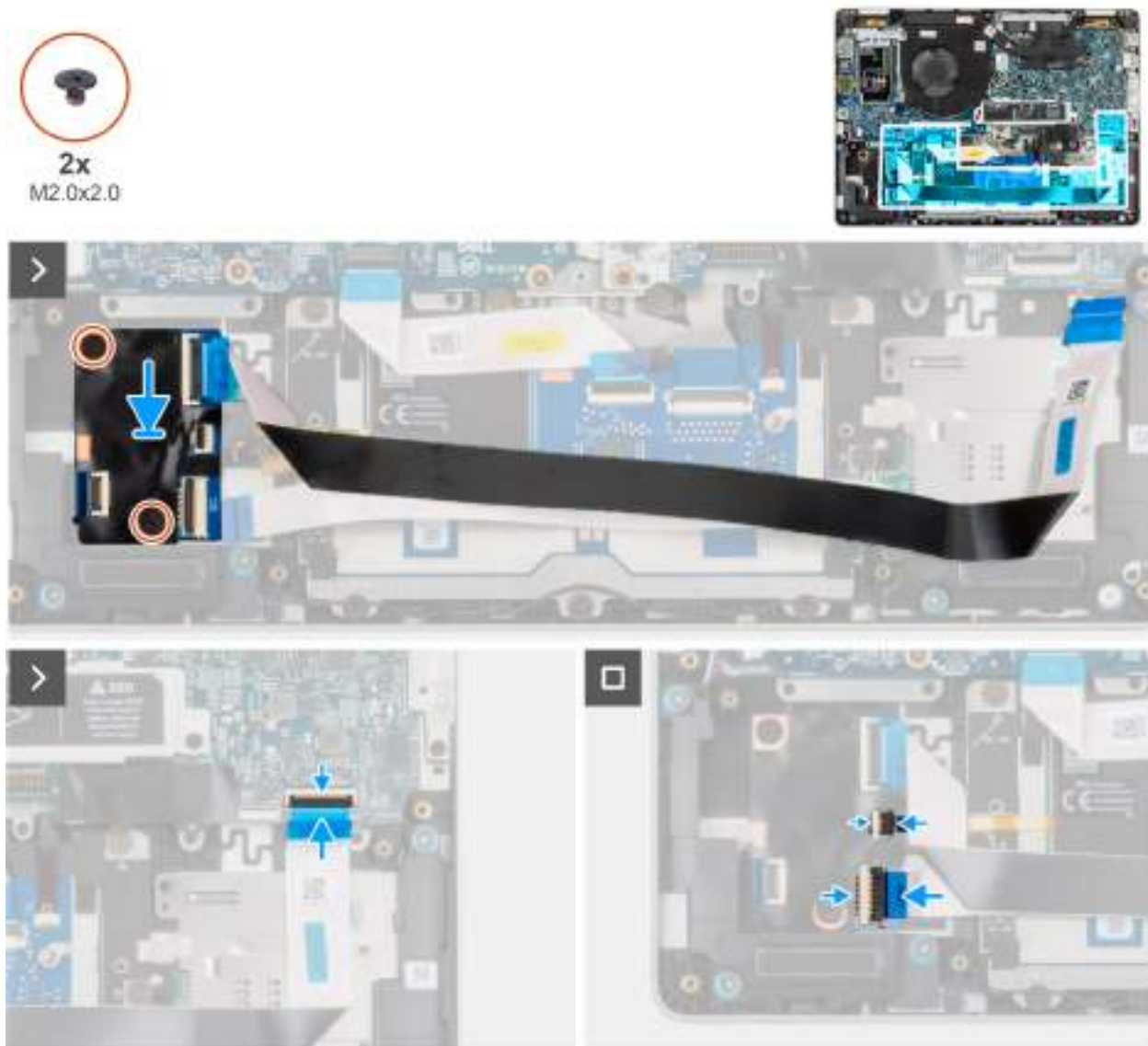
Obrázek 23. Montáž dceřiné desky USH
