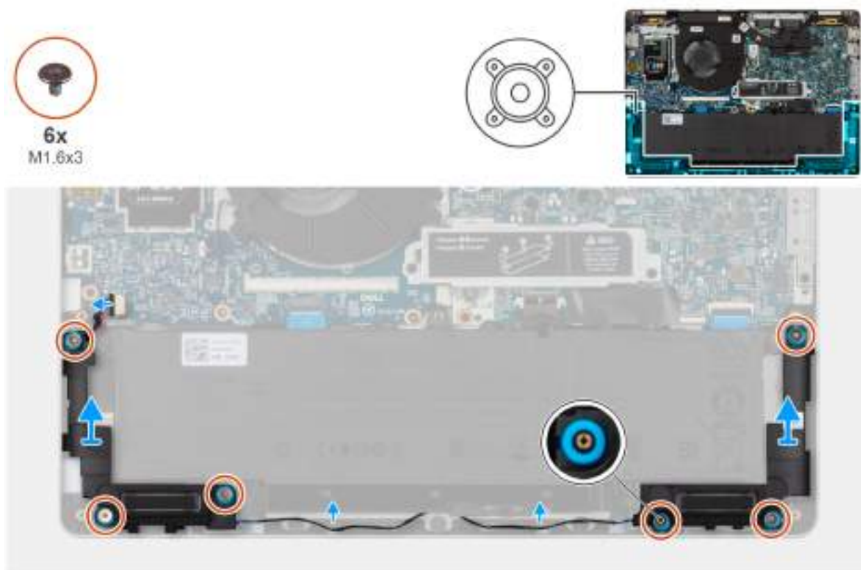
Obrázek 17. Demontáž reproduktorů
