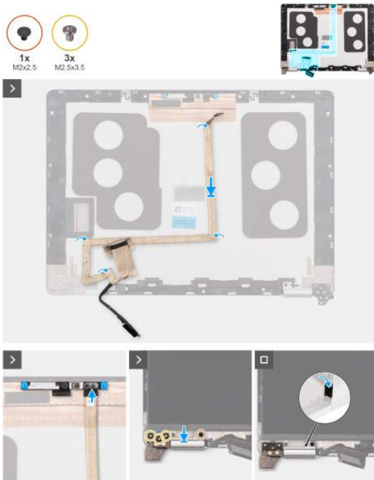
Obrázek 58. Vložení kabelu displeje
