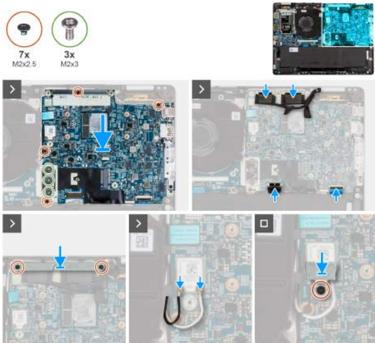
Obrázek 35. Montáž základní desky
