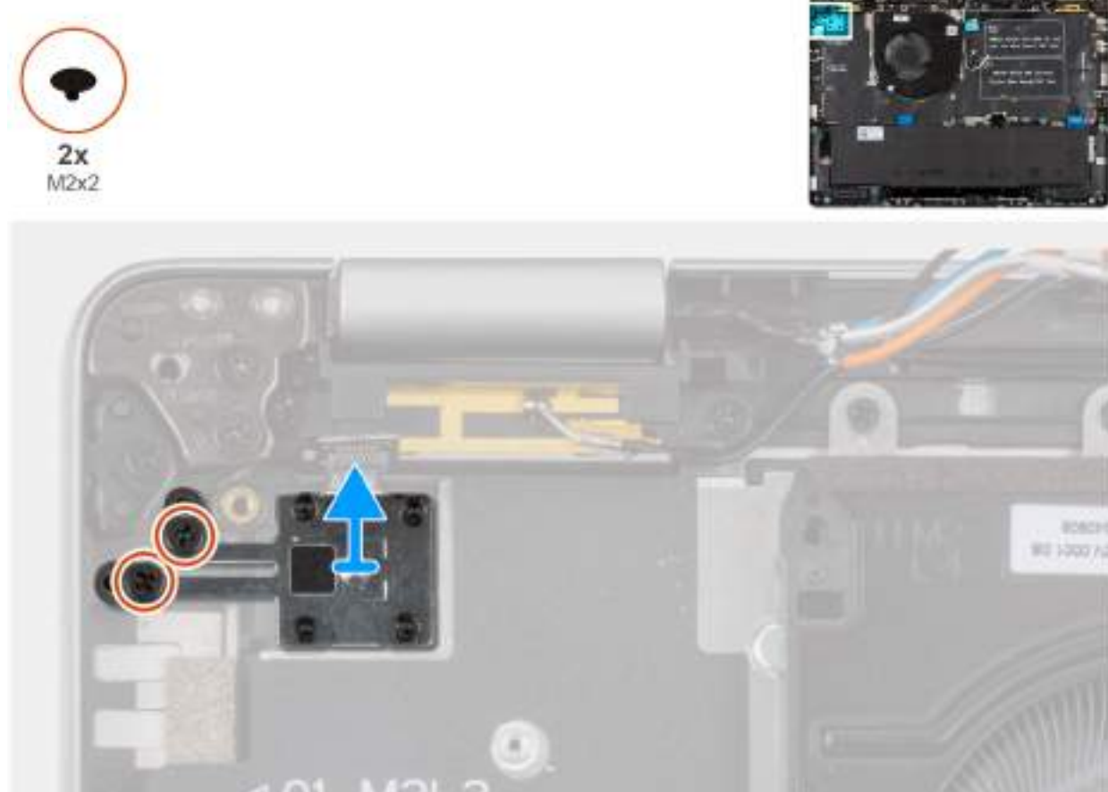
Obrázek 38. Demontáž vypínače s volitelnou čtečkou otisků prstů
