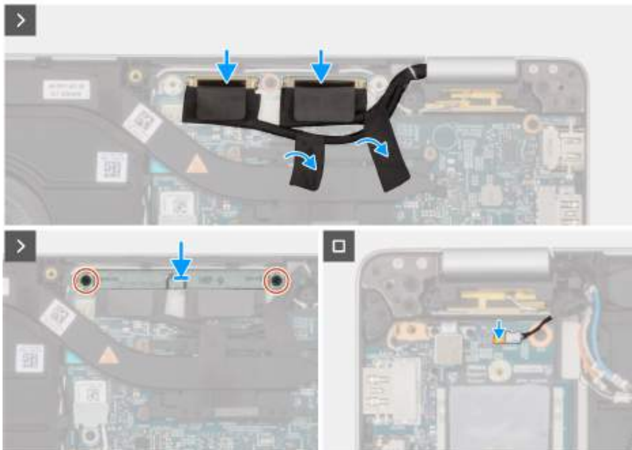
Obrázek 47. Montáž sestavy displeje
