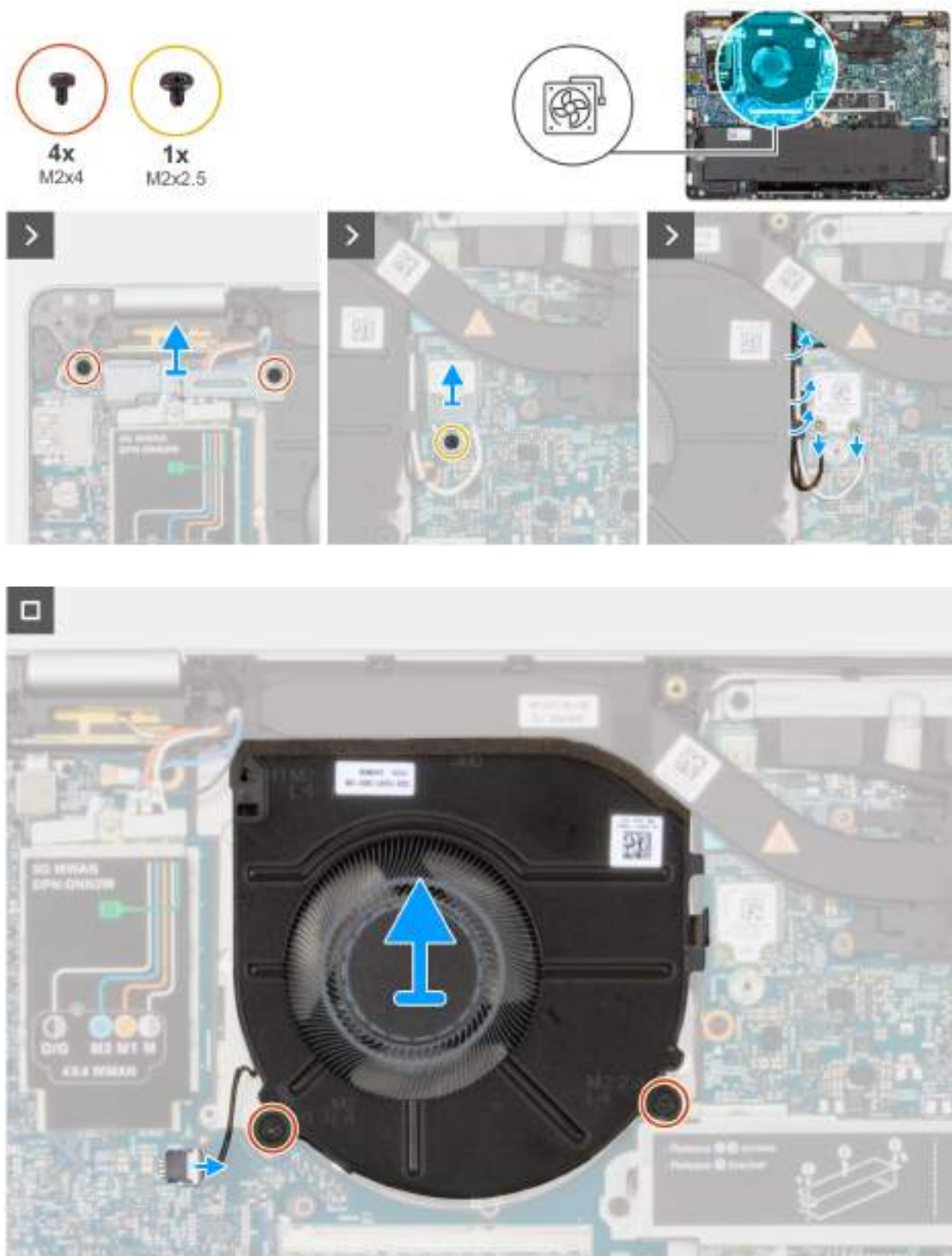
Obrázek 19. Demontáž ventilátoru
