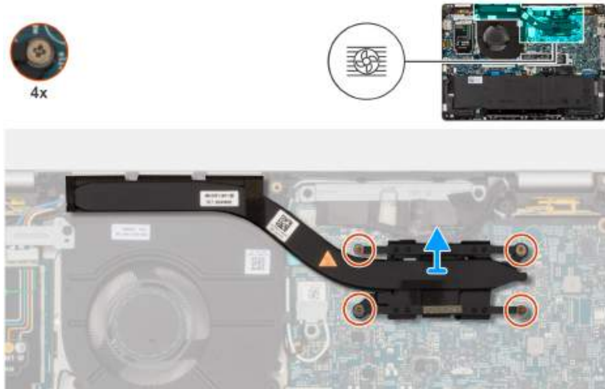
Obrázek 30. Demontáž chladiče
