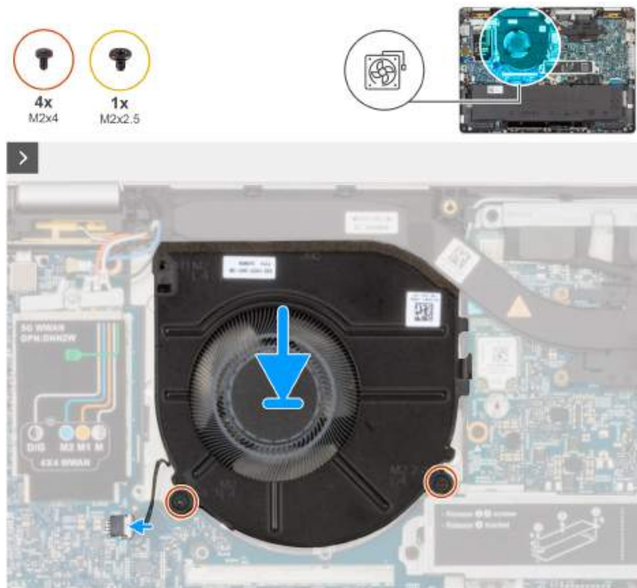
Obrázek 20. Instalace ventilátoru
